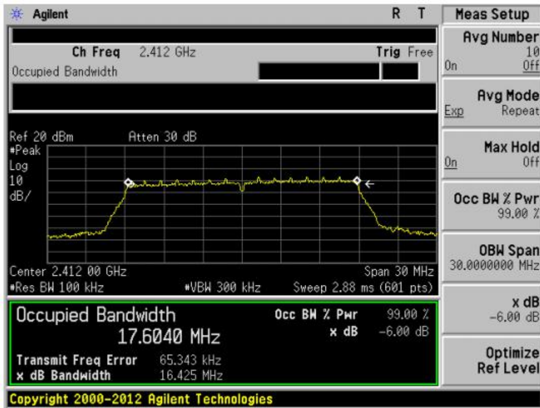
802.11n 20-2412MHz
