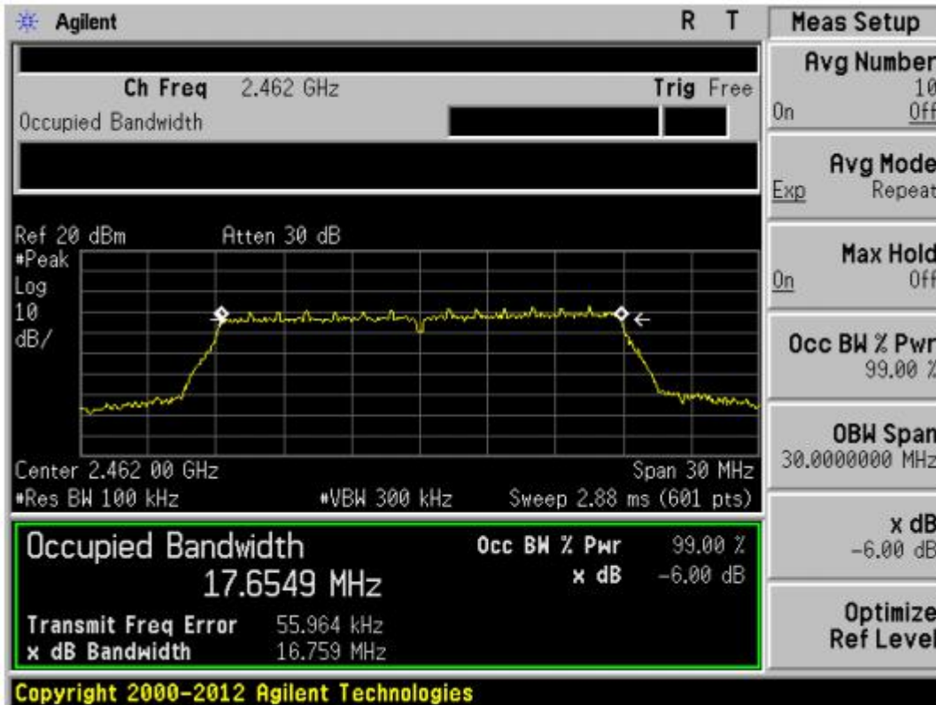
802.11n 20-2462MHz
