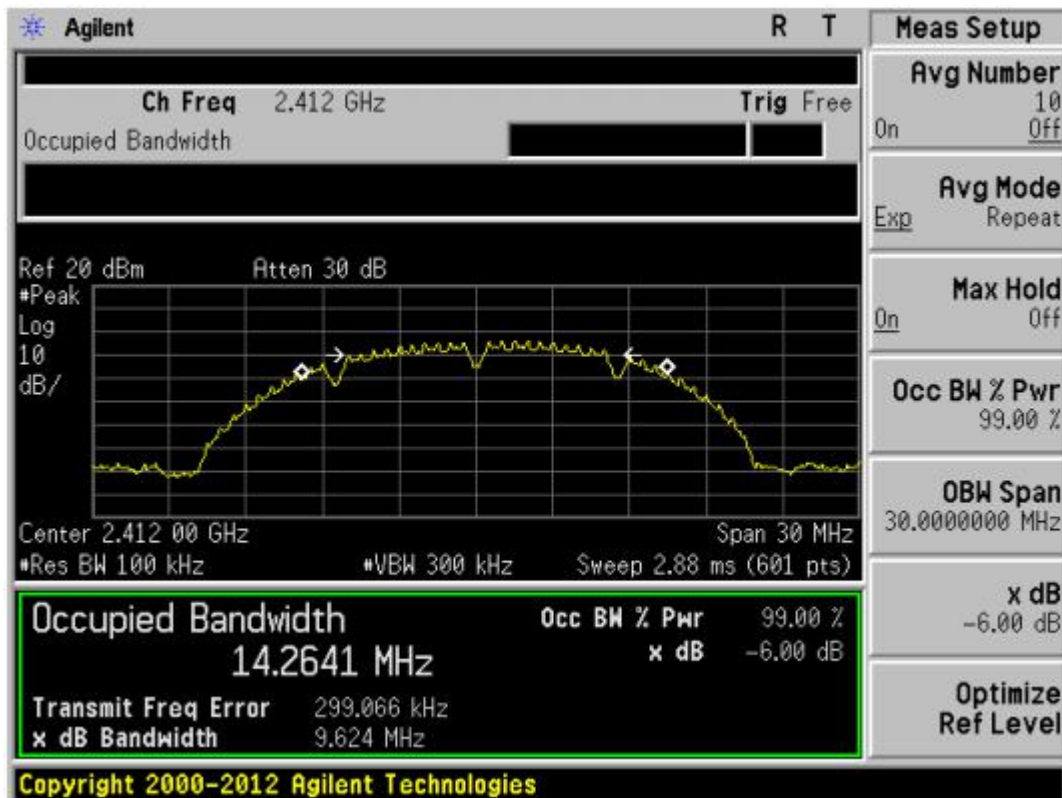
802.11b-CH2412MHZ
