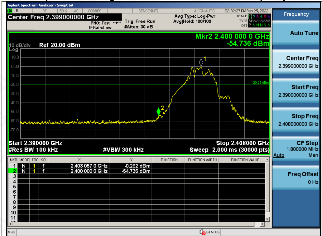
Test_Graph_GFSK_ANT1_2403_Lower Band Edge Emissions
