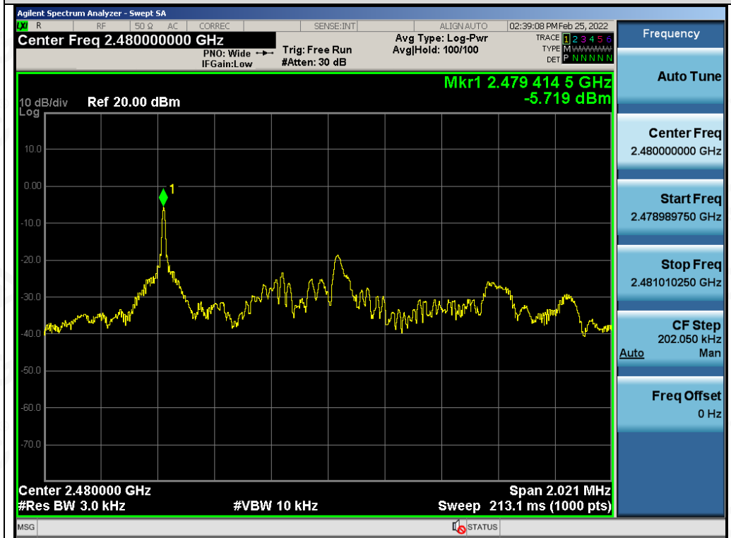
Test_Graph_GFSK_ANT1_2480_2Mbps_PSD
