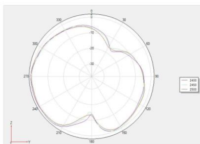
Phi 90 2D图
