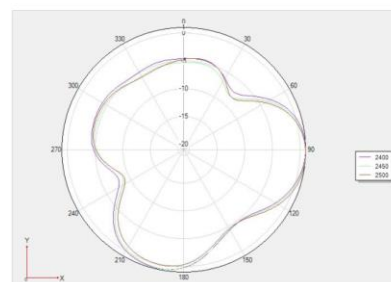
Theta 90 2D图
