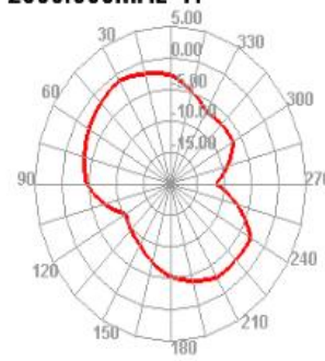
2500.000MHz H
