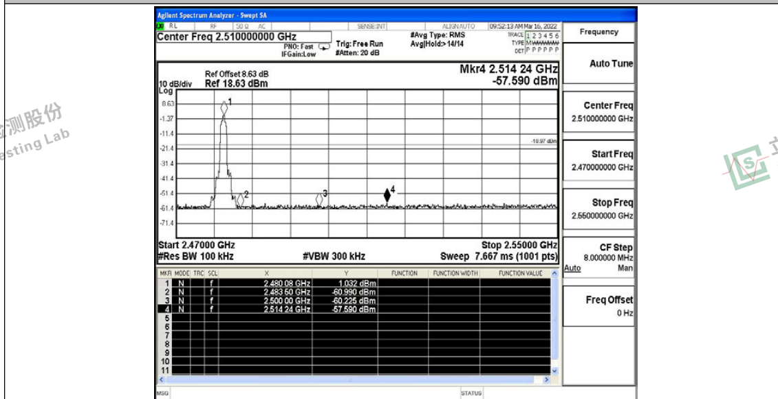
3DH5_Ant1_Low_Hop_2402
