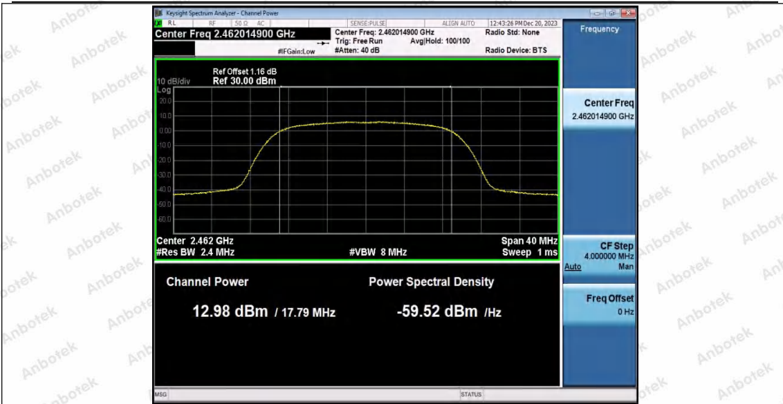
11N20SISO_WiFi_1_2462
