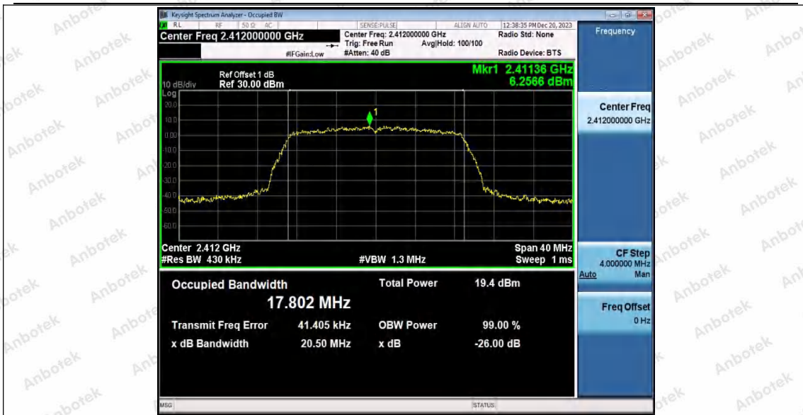
11N20SISO_WiFi_1_2412
