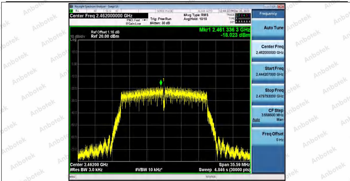
11N20SISO_WiFi_1_2462
