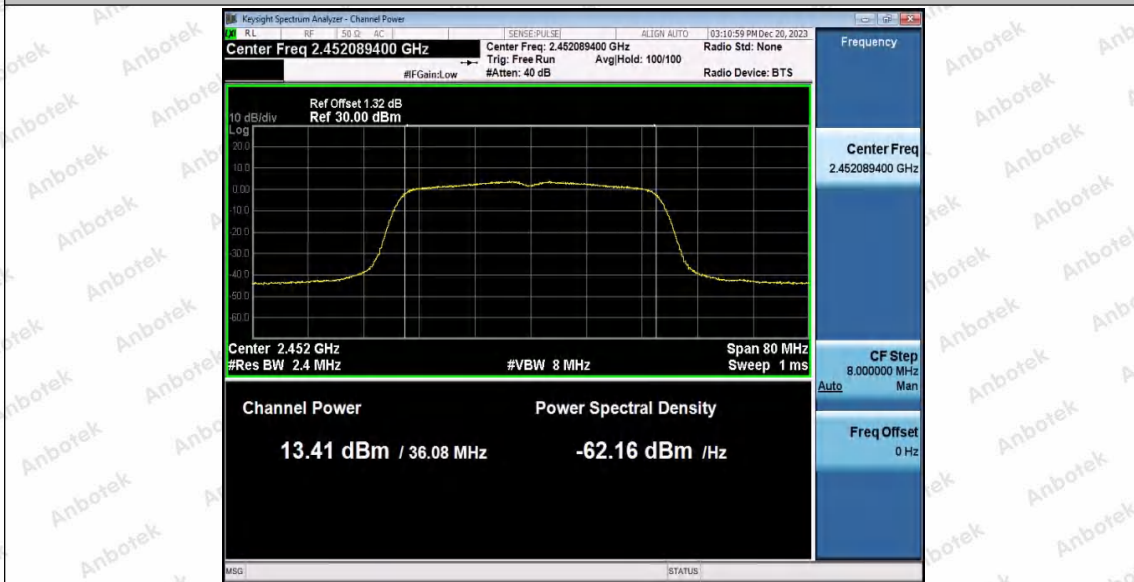
11N40SISO_WiFi_1_2452
