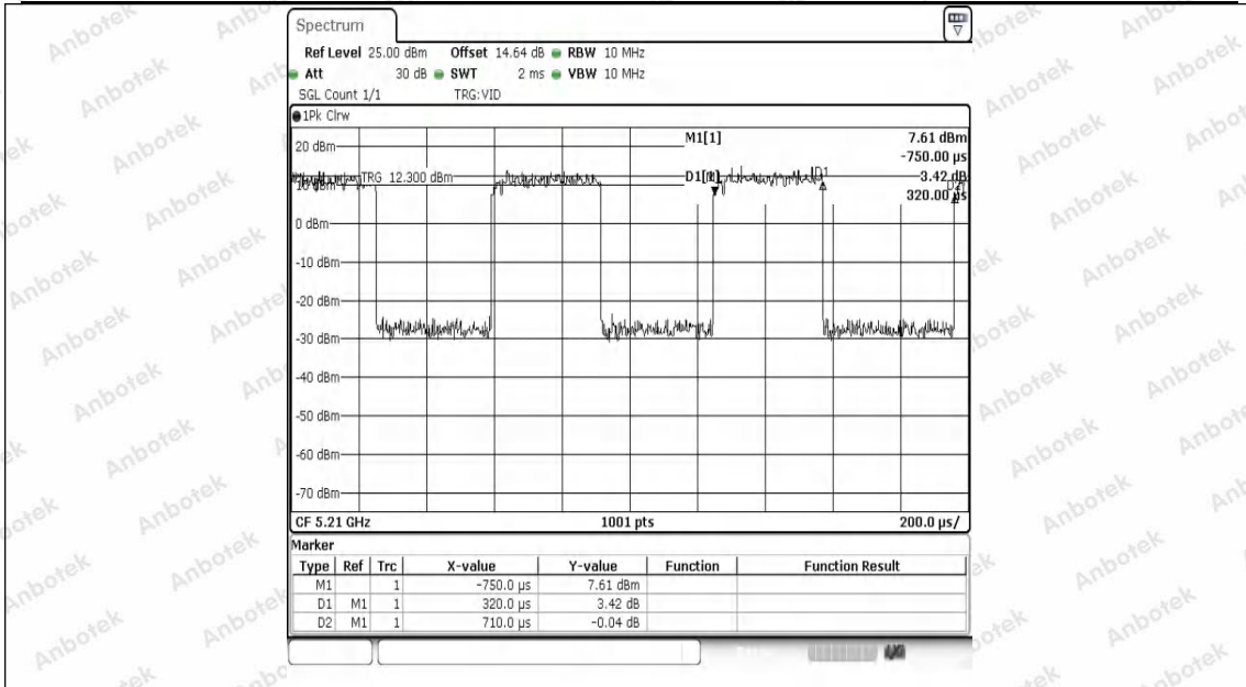
NTNV-11AC80SISO-Ant1-5210
