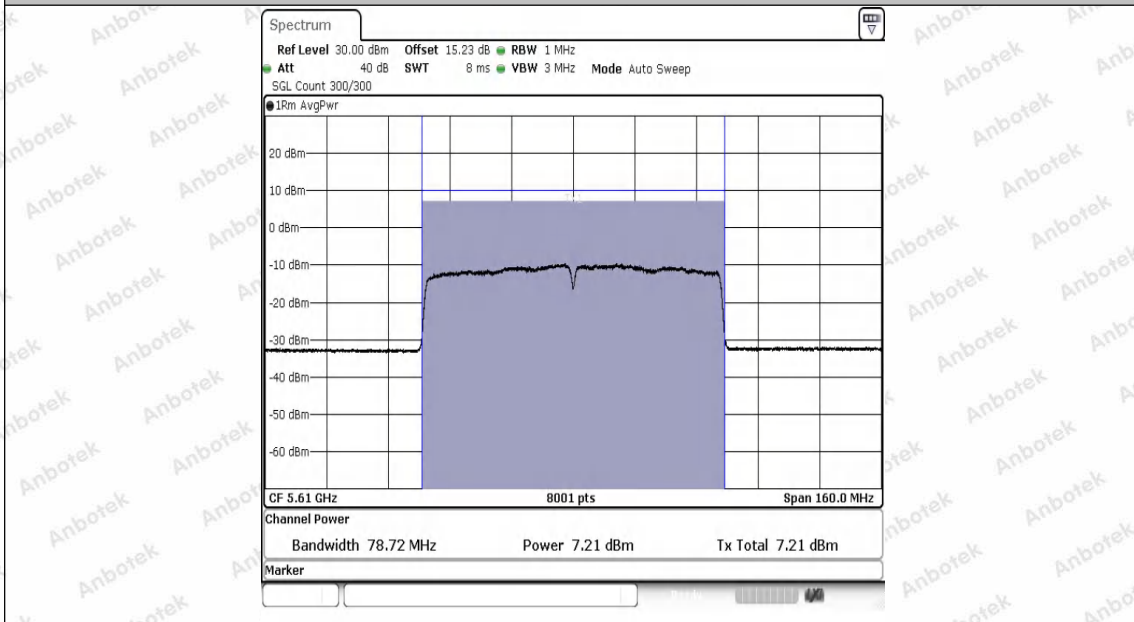
11AC80SISO-Ant1-5610-PASS
