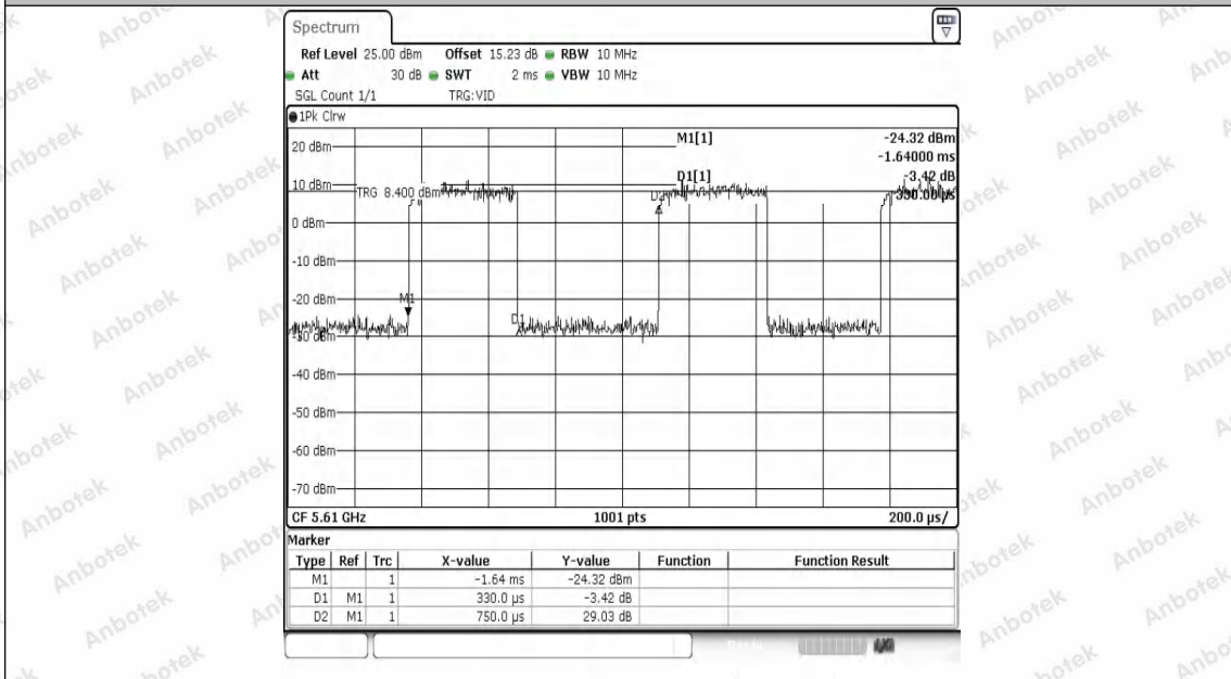
NTNV-11AC80SISO-Ant1-5610
