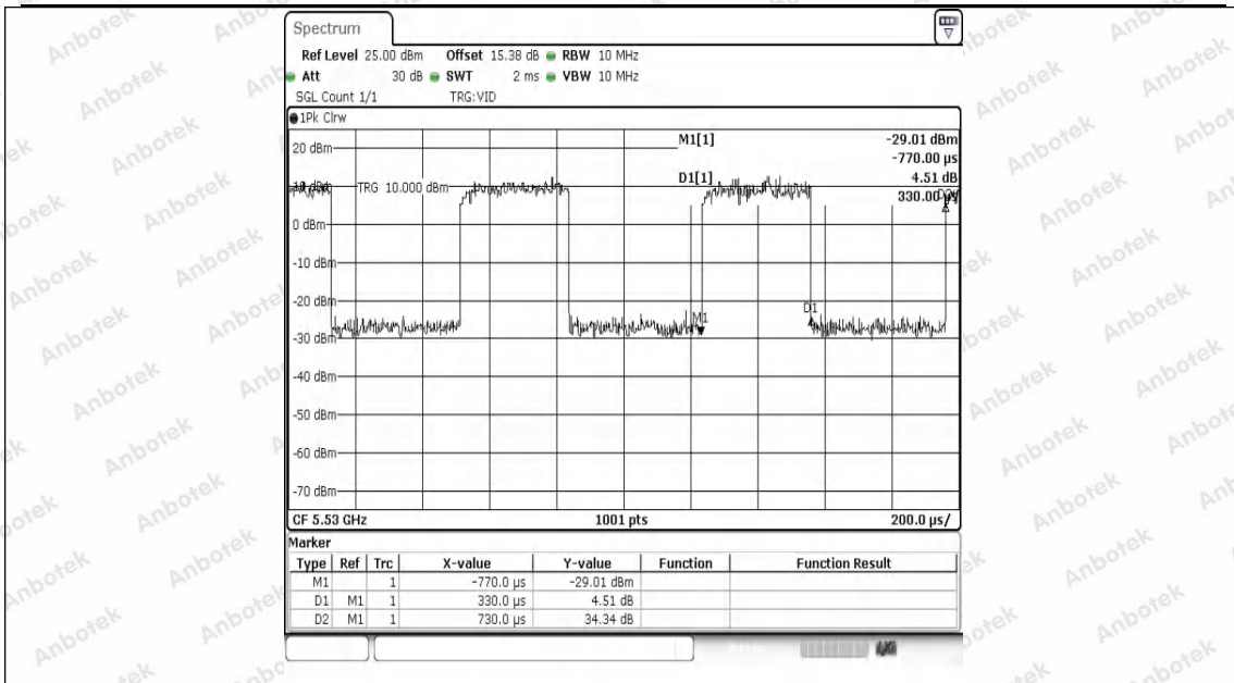
NTNV-11AC80SISO-Ant1-5530
