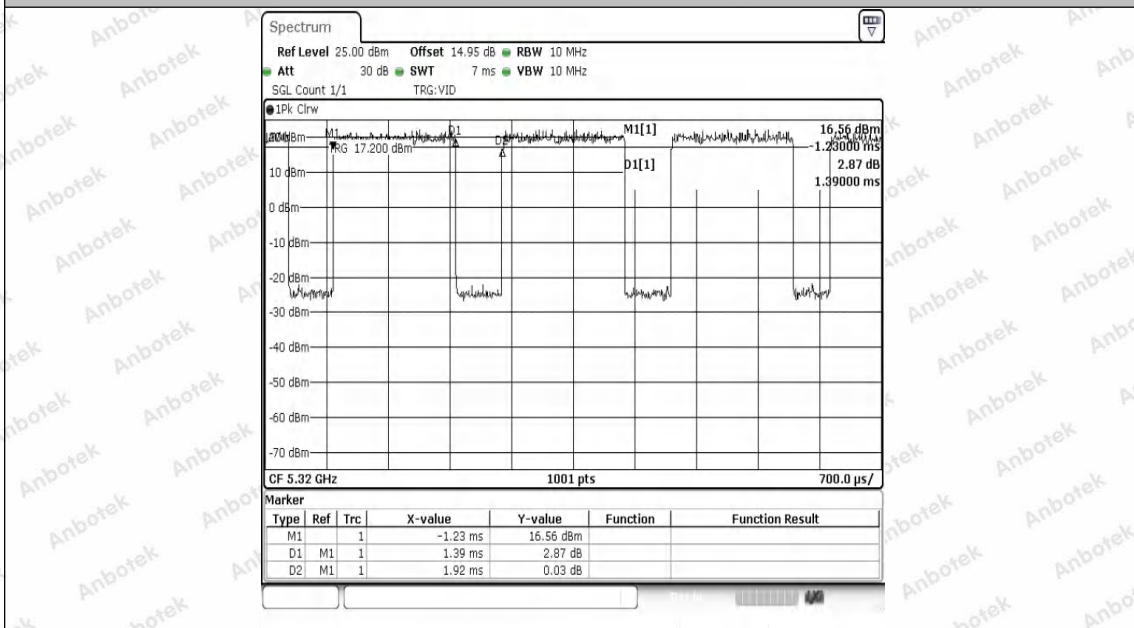
NTVN-11A-Ant1-5320
