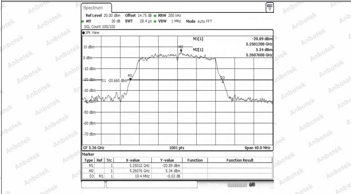
11A-Ant1-5260
