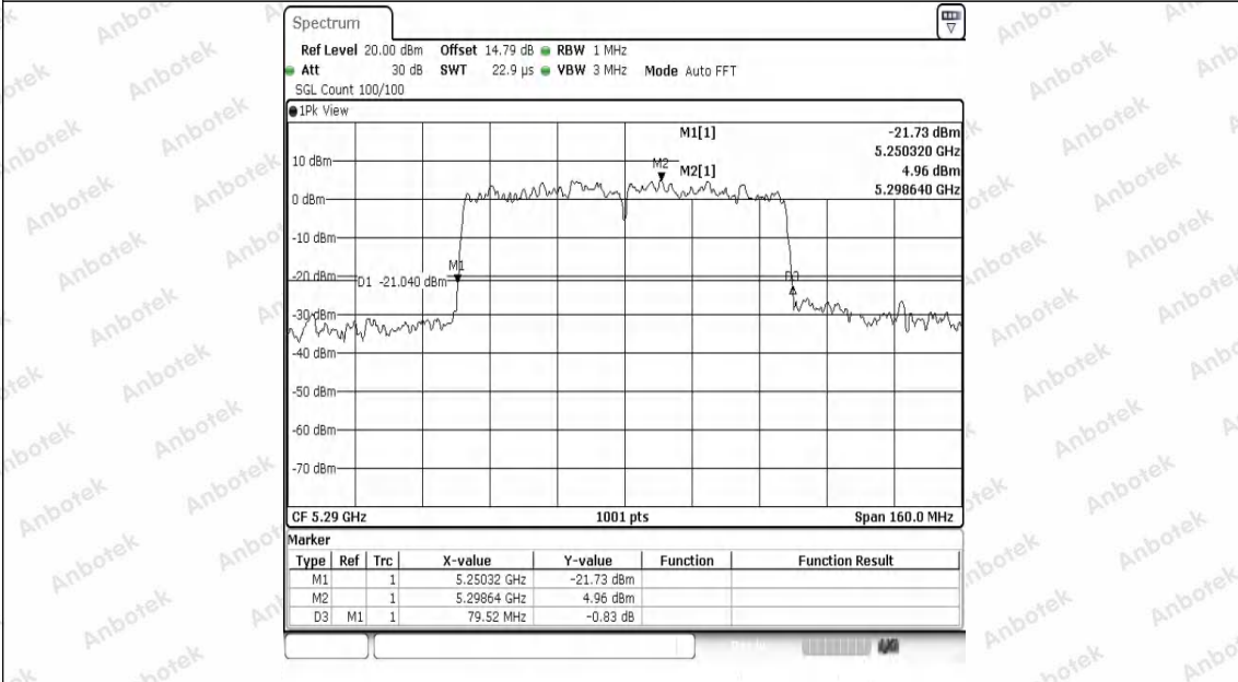
11AC80SISO-Ant1-5290
