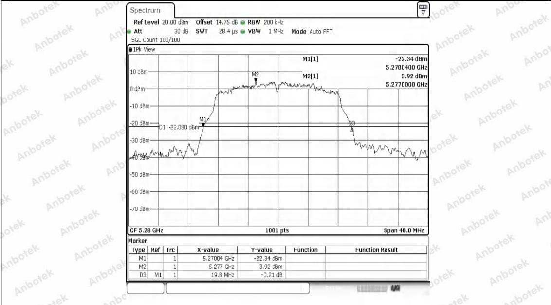
11A-Ant1-5280
