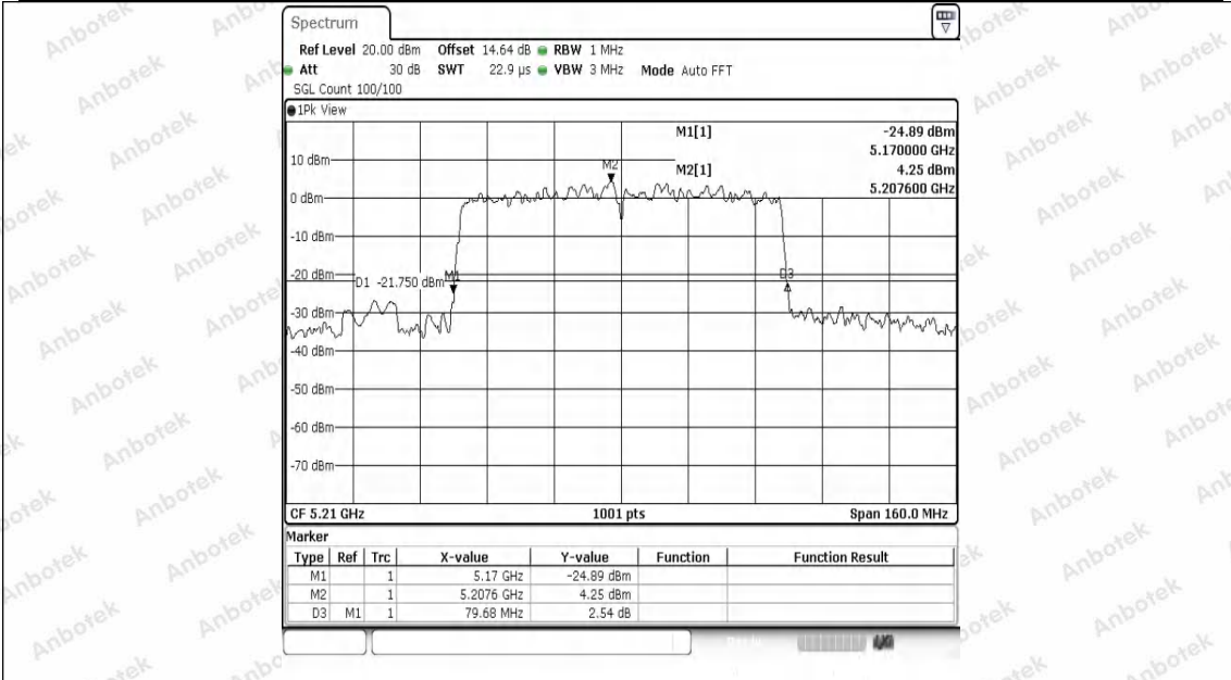
11AC80SISO-Ant1-5210
