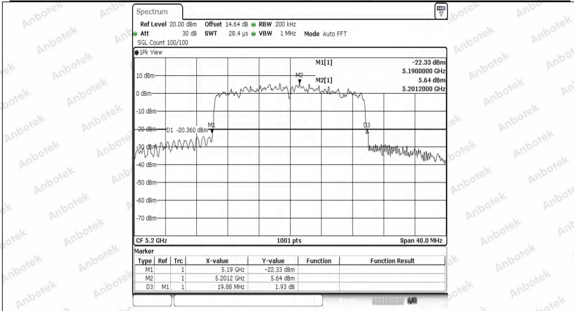
11AX20SISO-Ant1-5200
