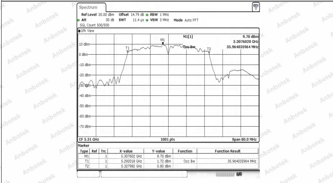
11N40SISO-Ant1-5310
