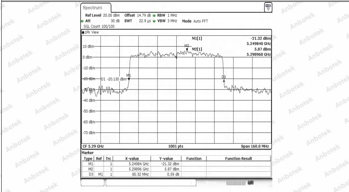
11AX80SISO-Ant1-5290
