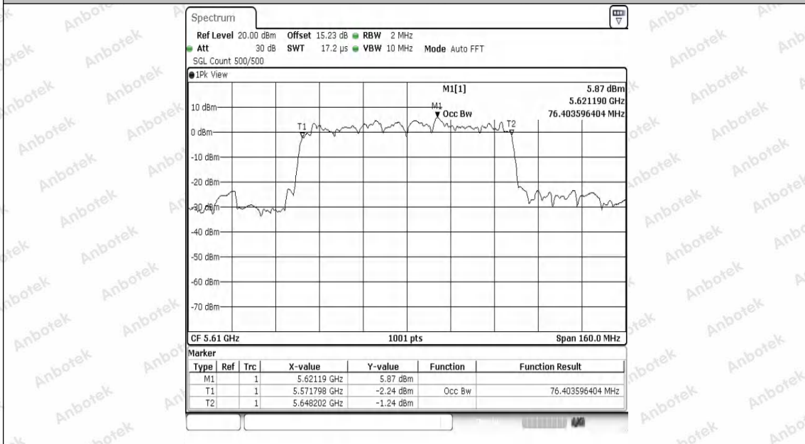
11AC80SISO-Ant1-5610
