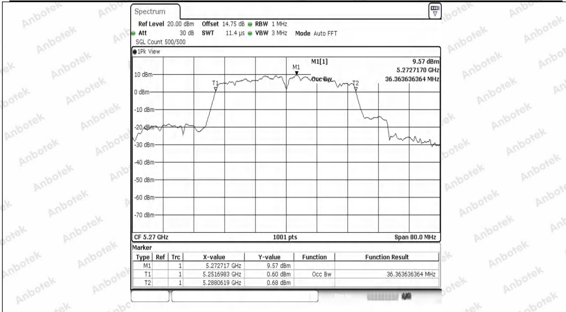
11N40SISO-Ant1-5270
