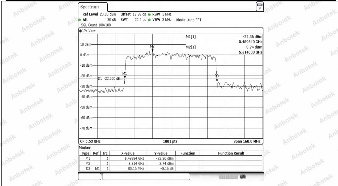
11AX80SISO-Ant1-5530
