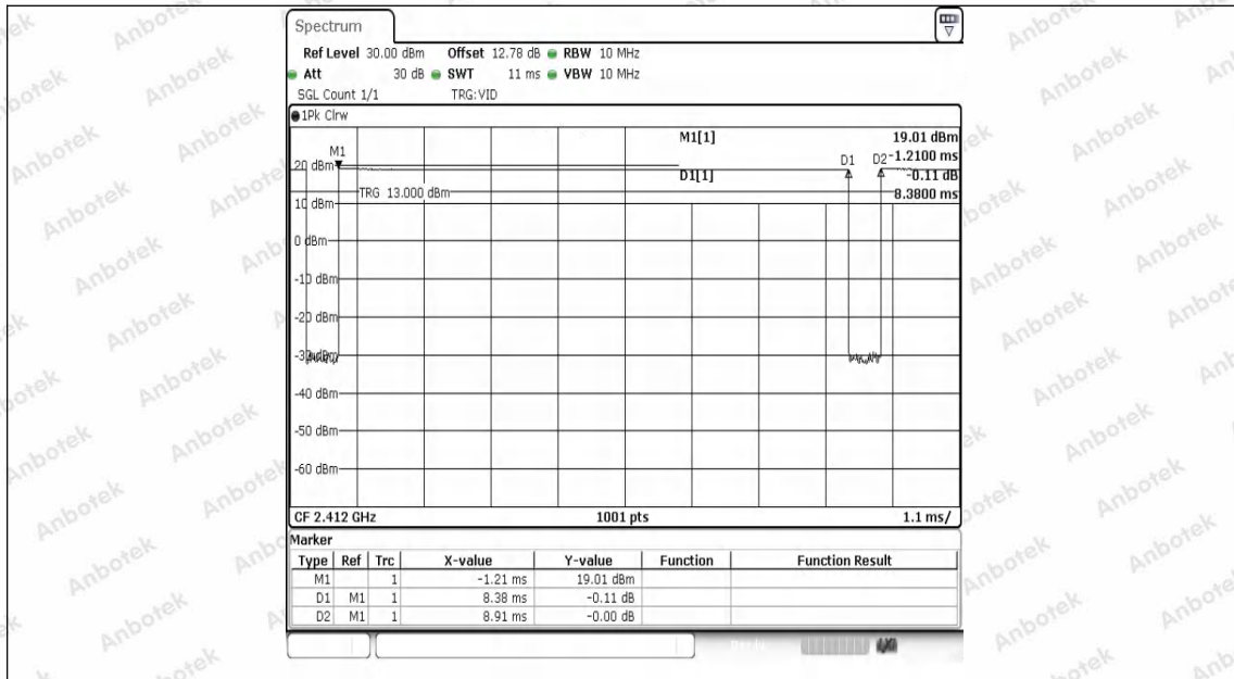
NTVN-11B-Ant1-2412
