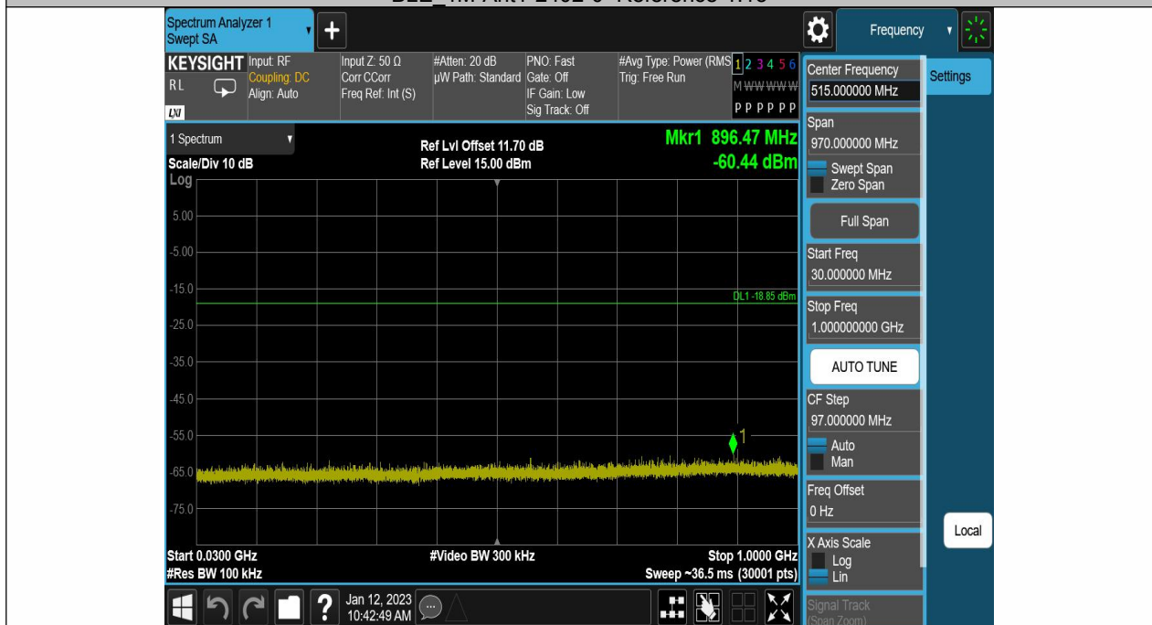
BLE_1M-Ant1-2402-30~1000-1.15
