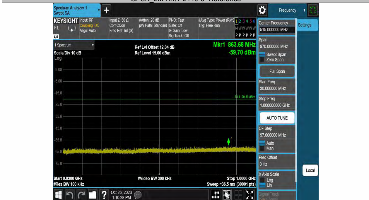
GFSK 2M-Ant1-2440-30~1000
