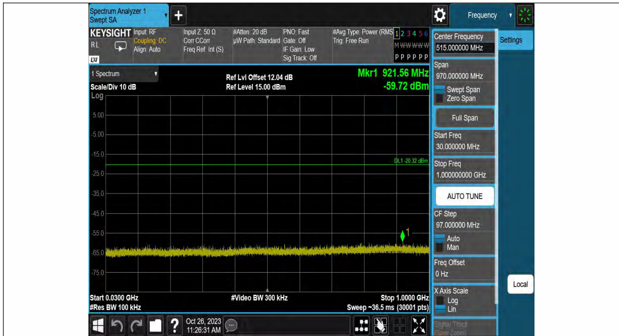
GFSK_1M-Ant1-2440-30~1000
