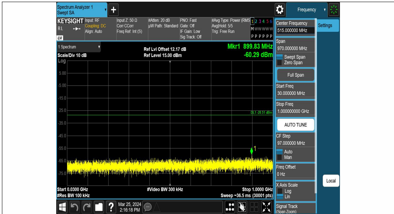
BLE_2M-Ant1-2478-30~1000-PASS
