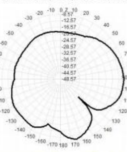
433.0MHz Total( E2-YZ), Max=- 2.13dBi
