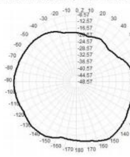
433.0MHz Total( E1-XZ), Max=- 2.45dBi
