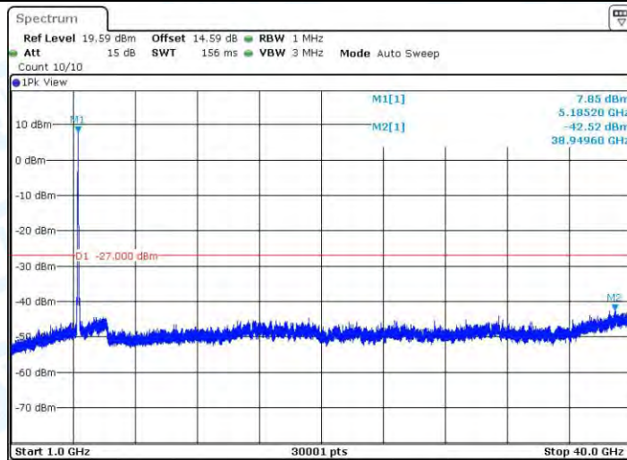
11AC40MIMO_Ant2_5190_1000~40000
