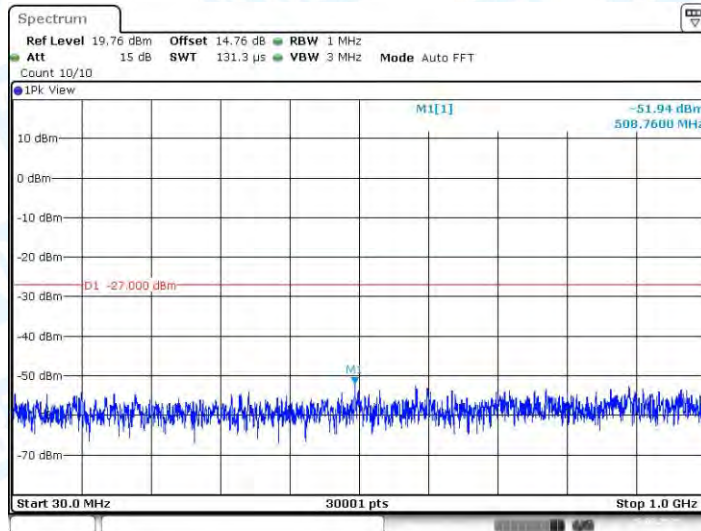
11AC20MIMO_Ant2_5240_30~1000
