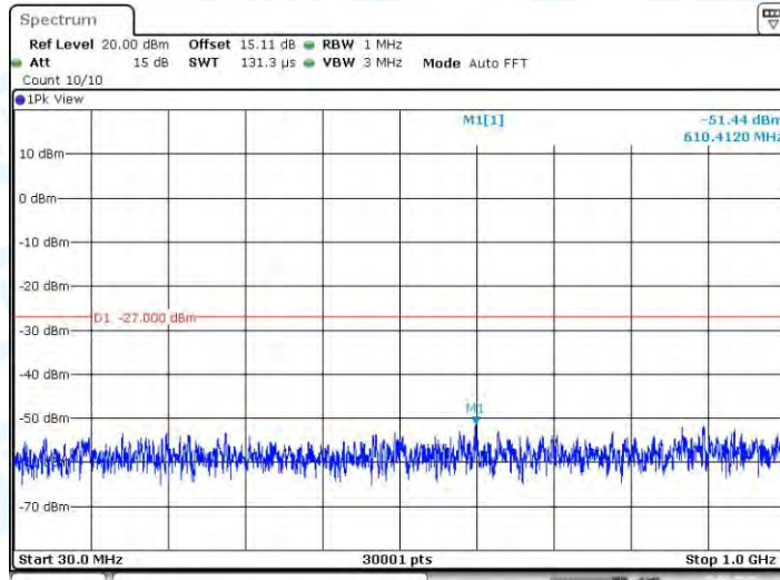
11N40MIMO_Ant2_5755_30~1000
