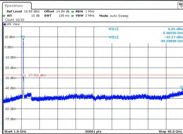
11AC80MIMO_Ant2_5290_1000~40000
