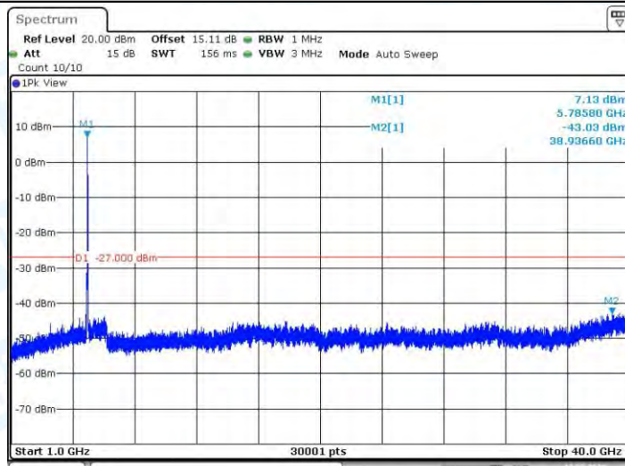
11N40MIMO_Ant2_5755_1000~40000
