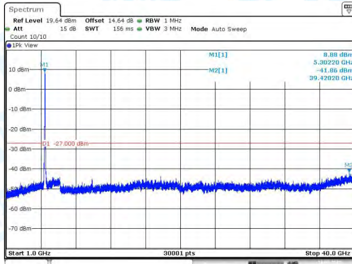
11AC40MIMO_Ant1_5310_1000~40000
