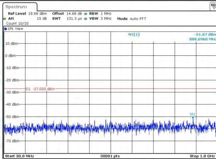
11AC40MIMO_Ant1_5230_30~1000
