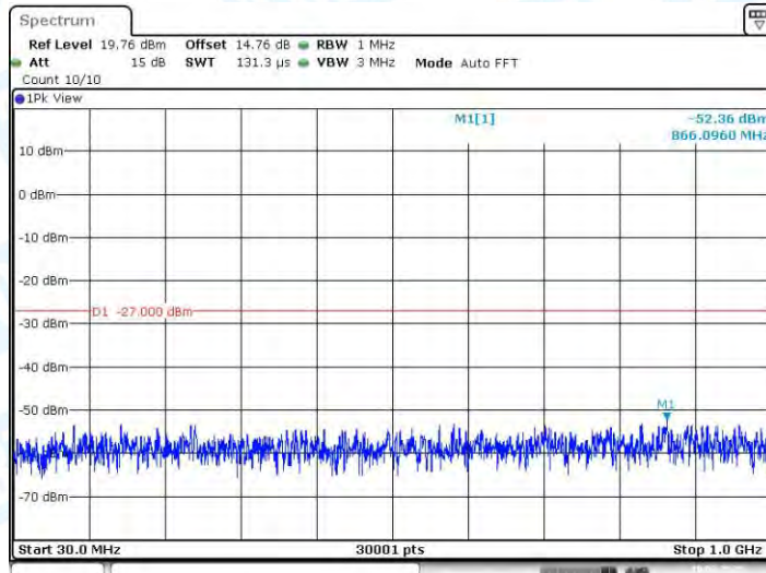
11N20MIMO_Ant2_5240_30~1000
