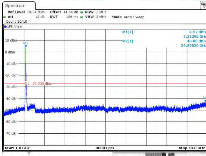
11AC80MIMO_Ant1_5210_1000~40000
