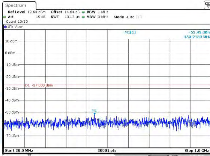
11AC40MIMO_Ant1_5310_30~1000
