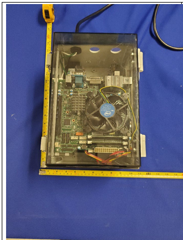
EUT – Top
