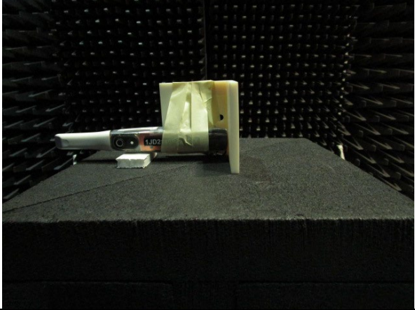
Horizontal EUT
