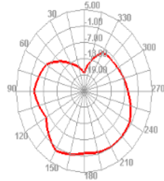
2450.000MHz E2
