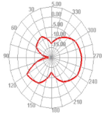
2450.000MHz E1
