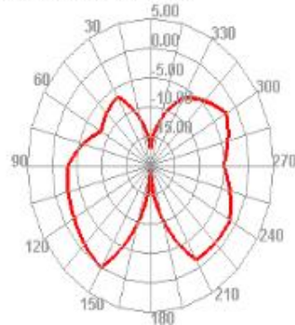
2450.000MHz H
