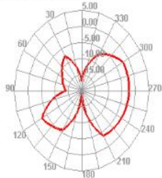
2450.000MHz
