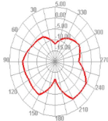
5150.000MHz H
