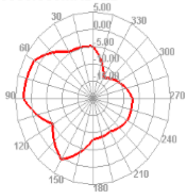
5150.000MHz E2
