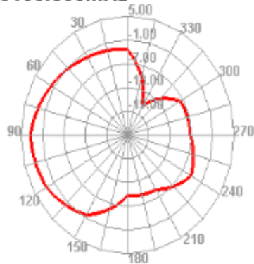
5150.000MHz H
