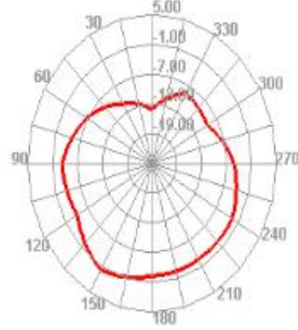
2400.000MHz E2
