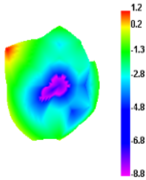
2450.000MHz E1
