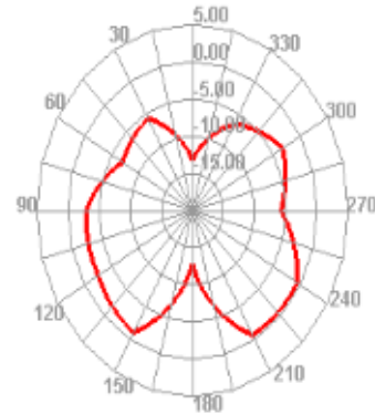
2450.000MHz E2
