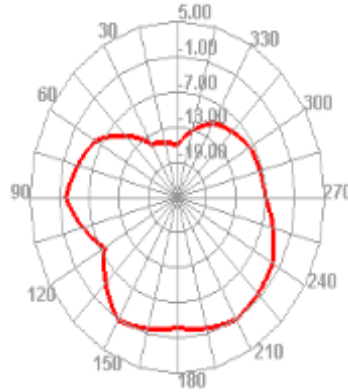
2500.000MHz E2
