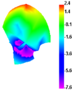
5150.000MHz E1
