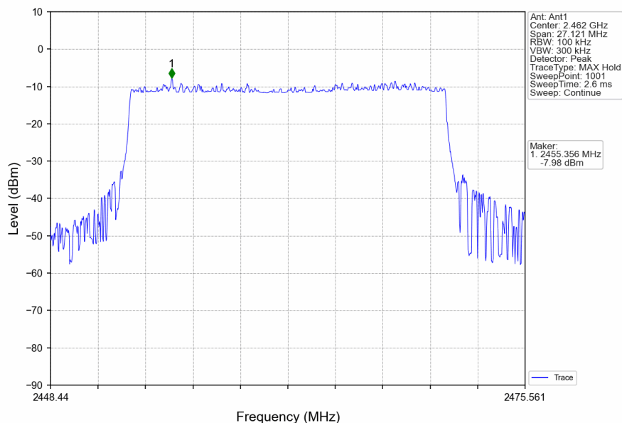
20M_HCH_2462MHz_Ant1_NTNV
