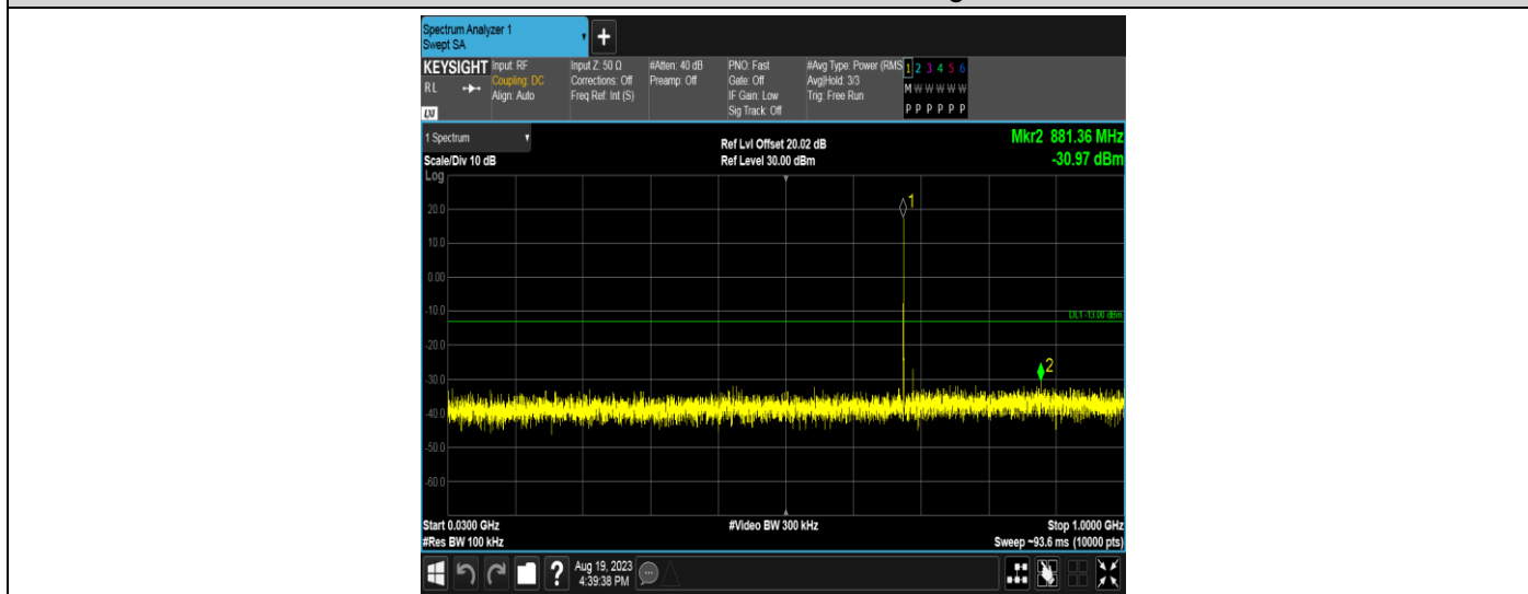
Band71-15MHz-QPSK-133397-1RB#0-Range1:30~1000MHz
