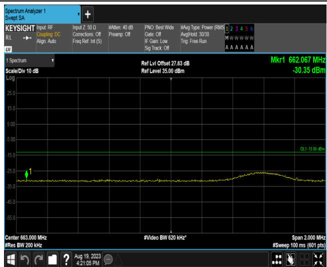
Band71-10MHz-QPSK-133172-1RB#49
