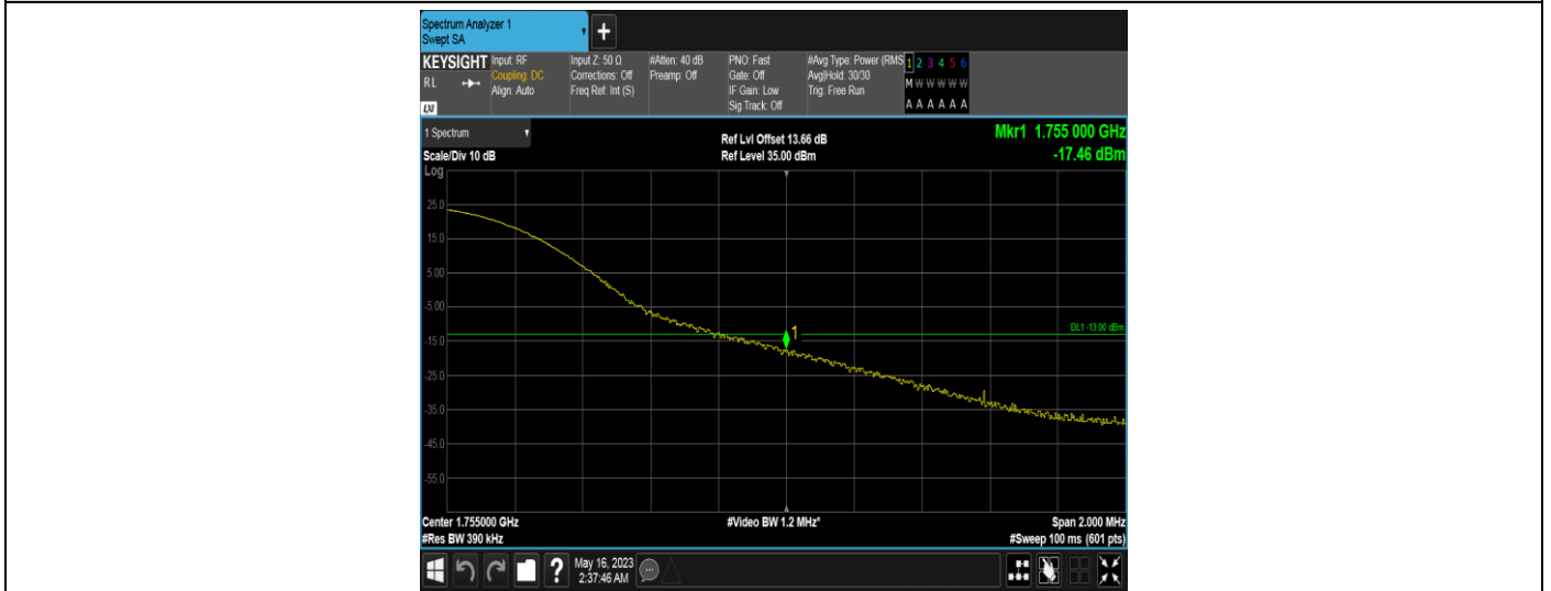
Band4-20MHz-QPSK-20300-1RB#99
