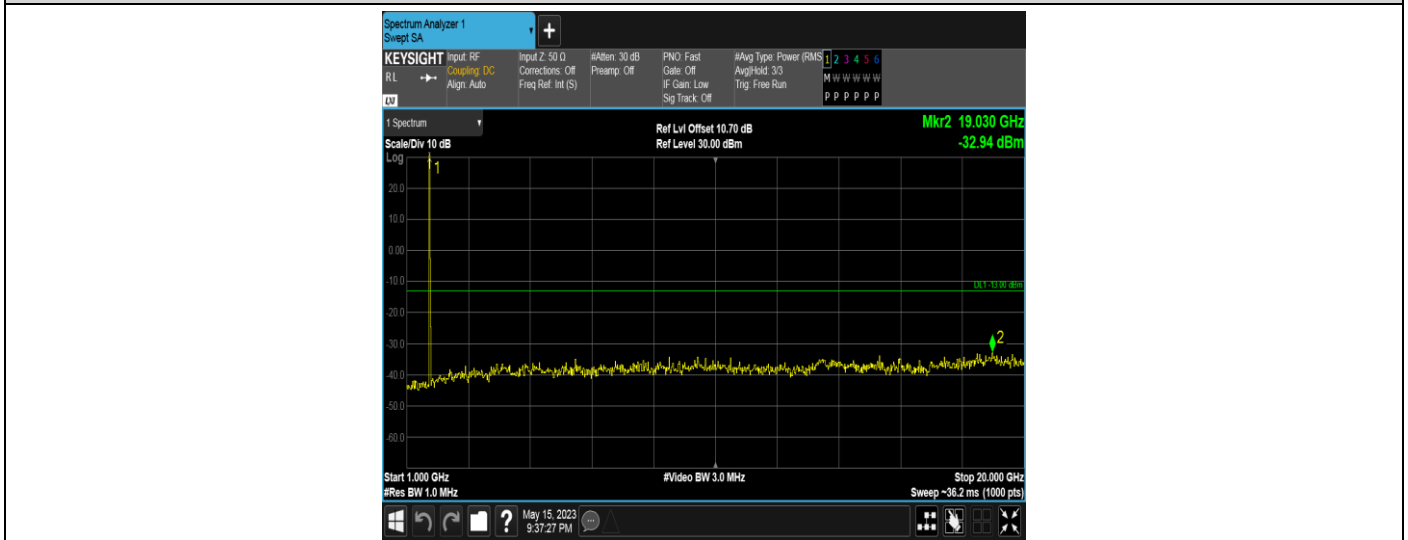
Band4-15MHz-QPSK-20025-1RB#0-Range2:1000~20000MHz
