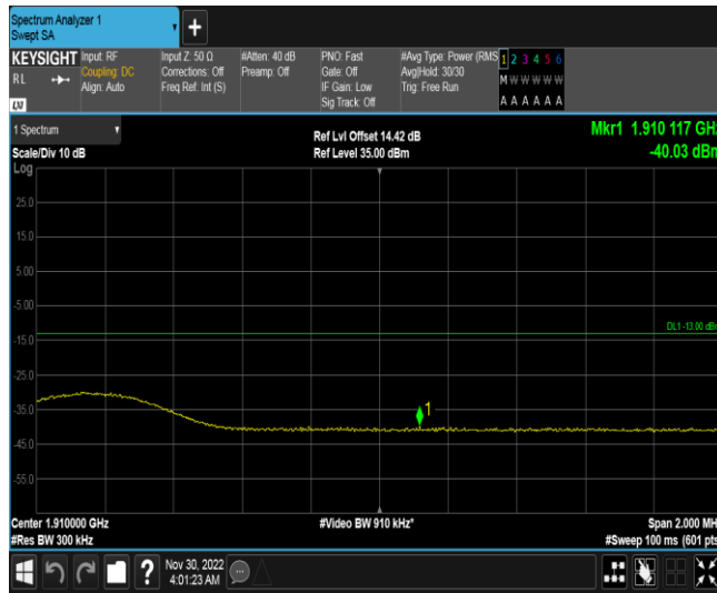
Band2-15MHz-16QAM-19125-1RB#74
