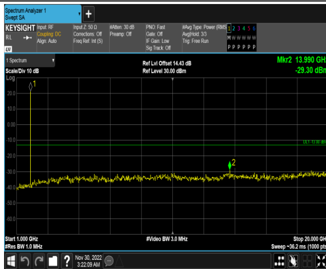
Band2-3MHz-16QAM-18615-1RB#0-Range2:1000~20000MHz
