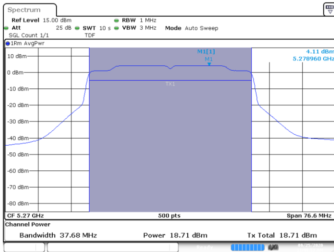
MIMO A-802.11ax-40MHz-Ch54-5270MHz-HE0
