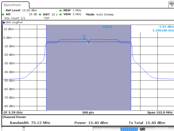
MIMO A-802.11ac-80MHz-Ch58-5290MHz-VHT0
