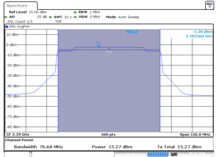
MIMO B-802.11ax-80MHz-Ch58-5290MHz-HE0
