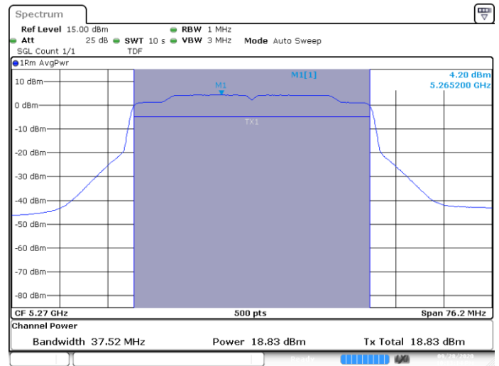
MIMO B-802.11ax-40MHz-Ch54-5270MHz-HE0
