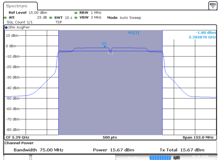
MIMO B-802.11ac-80MHz-Ch58-5290MHz-VHT0
