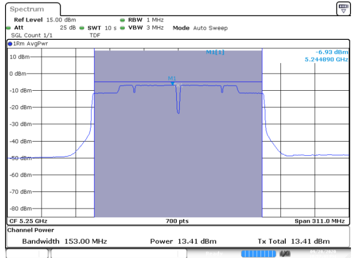
MIMO B-802.11ac-160MHz-Ch50-5250MHz-VHT0
