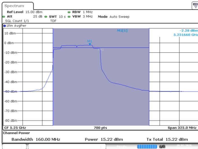
MIMO A-802.11ax-160MHz-Ch50-5250MHz-HE0
