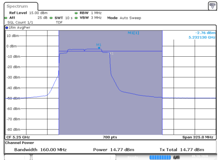
MIMO B-802.11ax-160MHz-Ch50-5250MHz-HE0
