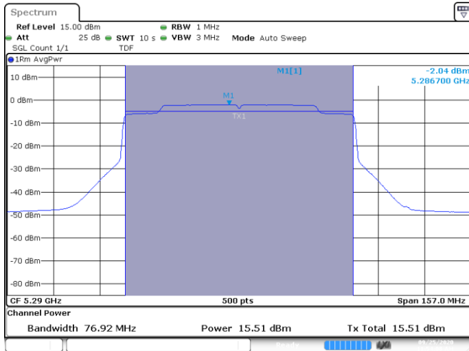
MIMO A-802.11ax-80MHz-Ch58-5290MHz-HE0
