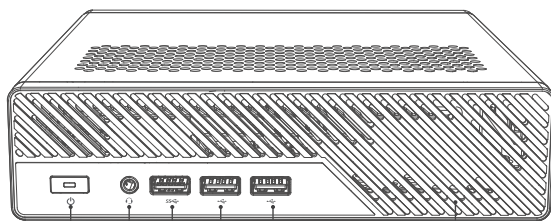
Netzschalter 01 3,5-mm-Kombibuchse 02 USB3.2 Anschluss 03 USB2.0 -Anschluss 04 Kühlkörperlöcher 05
