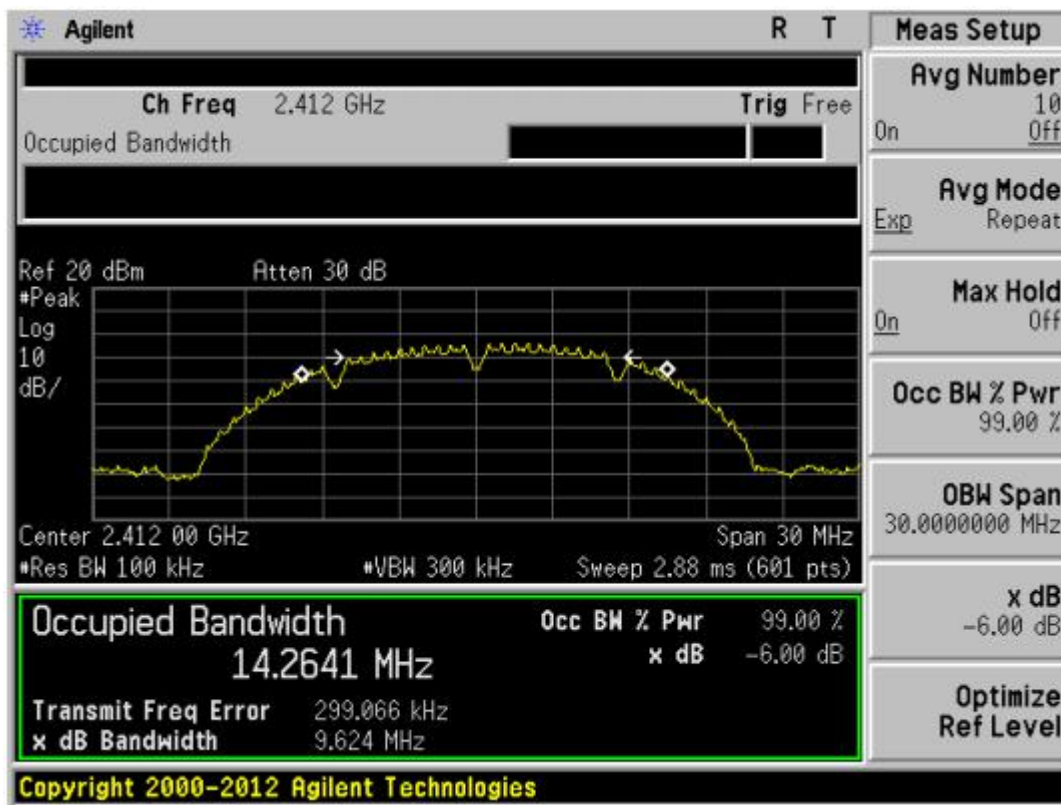
802.11b-CH2412MHZ
