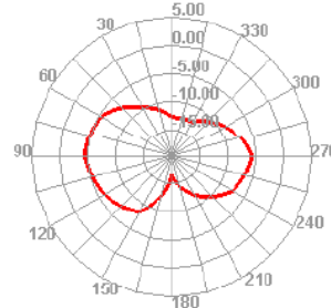
2480.000MHz E2
