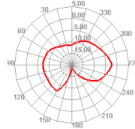
2470.000MHz E1
