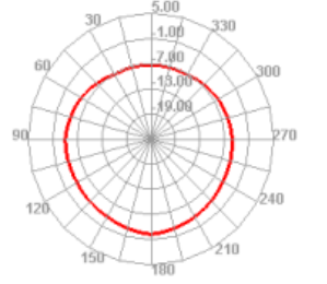
2470.000MHz H
