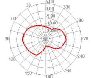
2440.000MHz E2
