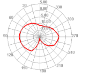
2470.000MHz E2
