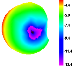
2480.000MHz
