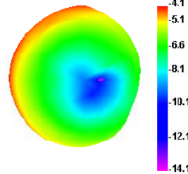
2440.000MHz
