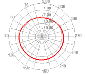
2440.000MHz H
