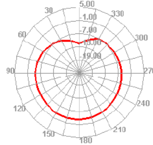
2480.000MHz H
