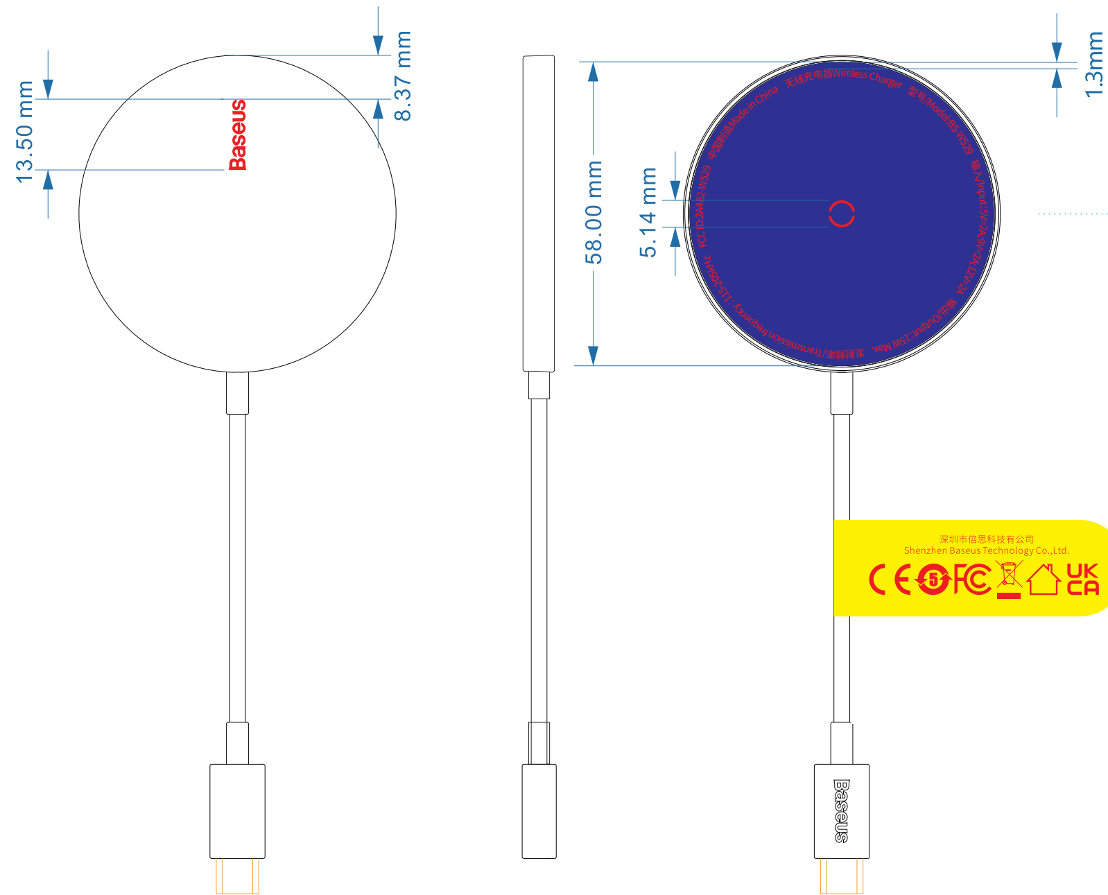
后视图
