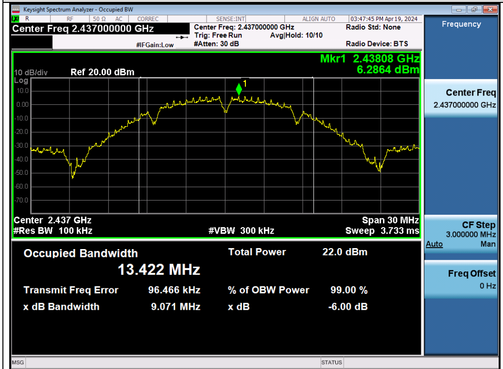
Test_Graph_802.11b_ANT1_2437_1Mbps_DTSSW
