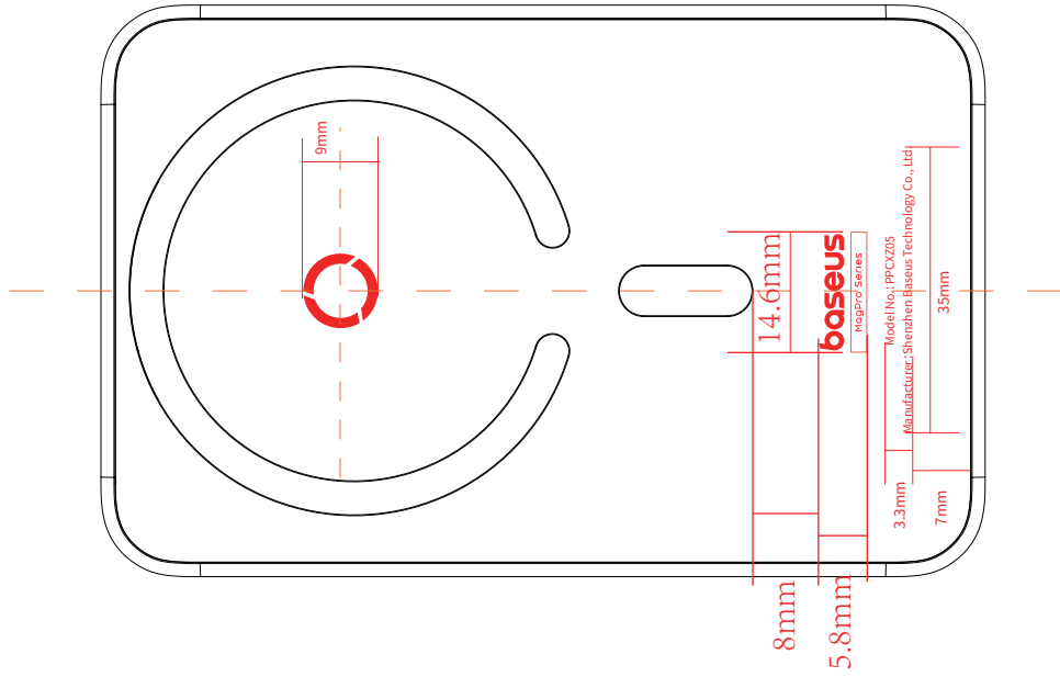
后视图
