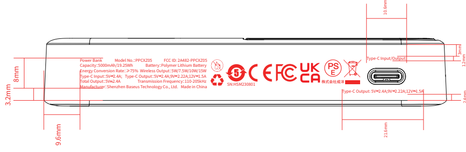
左视图
