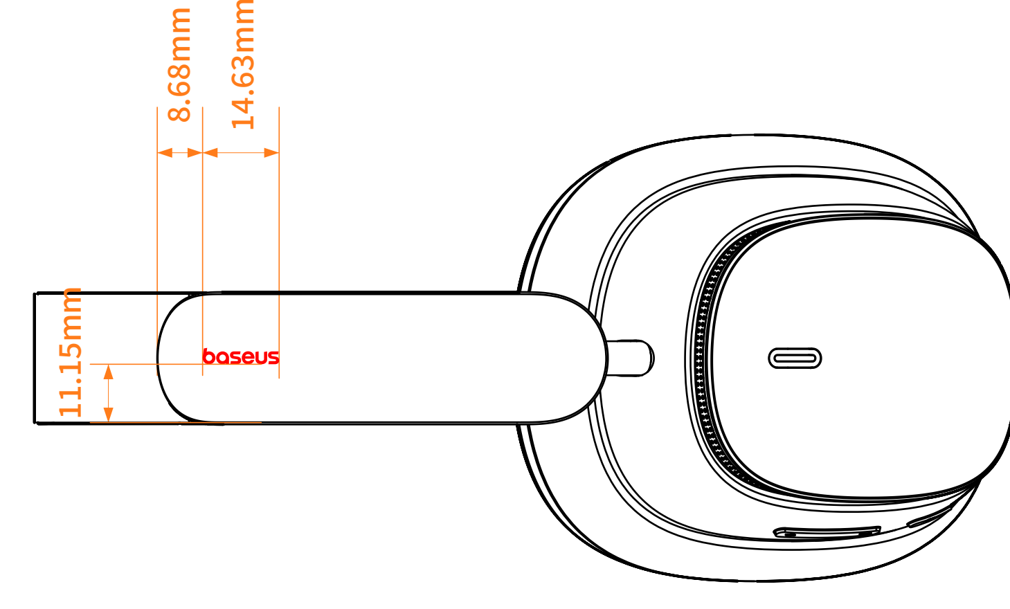
左视图
