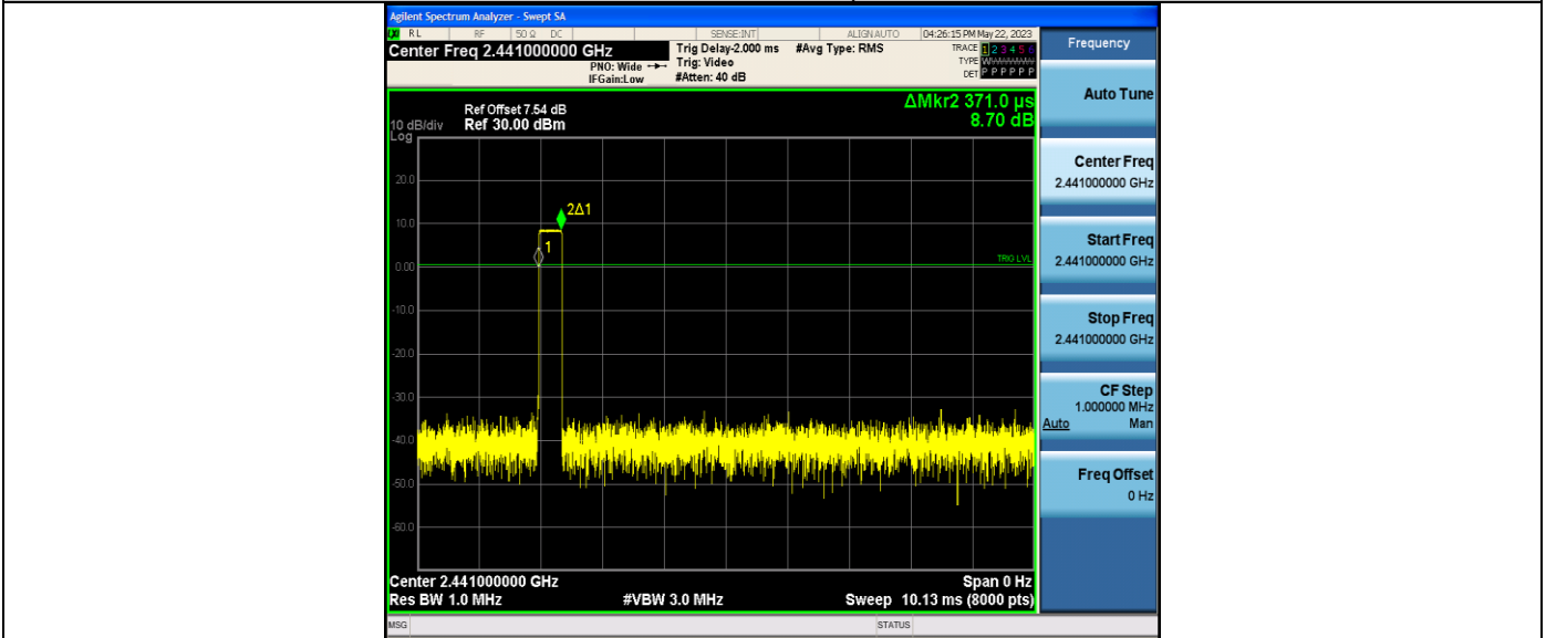
DH1_Ant1_Hop
