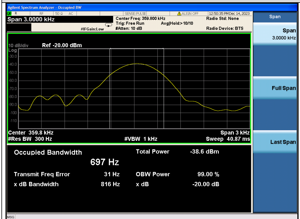
Test_Graph_ASK_Coil ANT_ 359.8kHz _ -20dB Bandwidth
