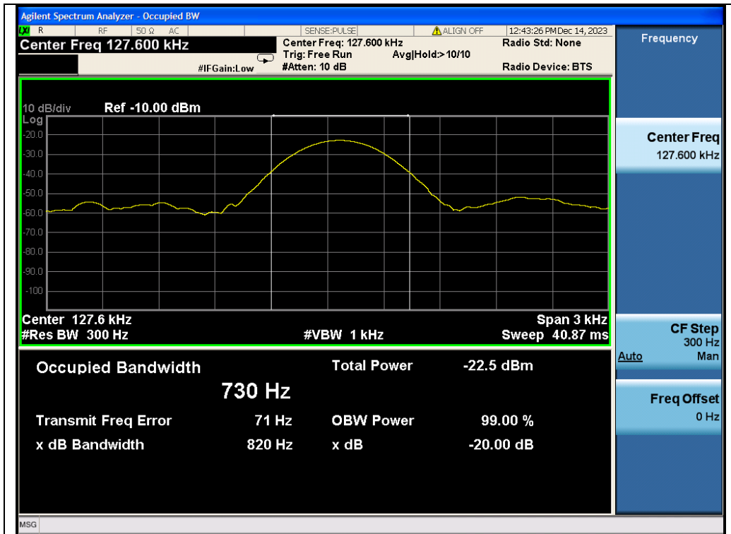
Test_Graph_ASK_Coil ANT_ 127.6kHz _ -20dB Bandwidth
