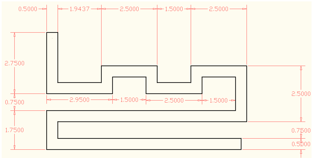
图 Normal Module Wiggle 天线 (Unit: mm)
