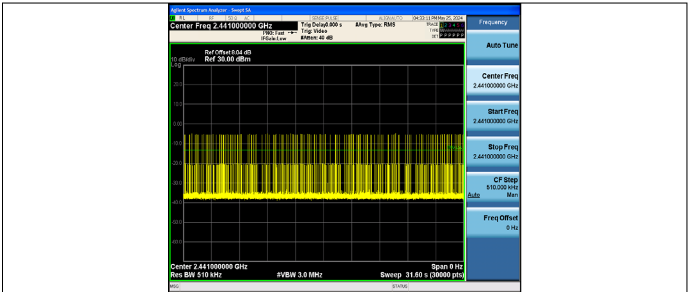
2DH5_Ant1_Hop
