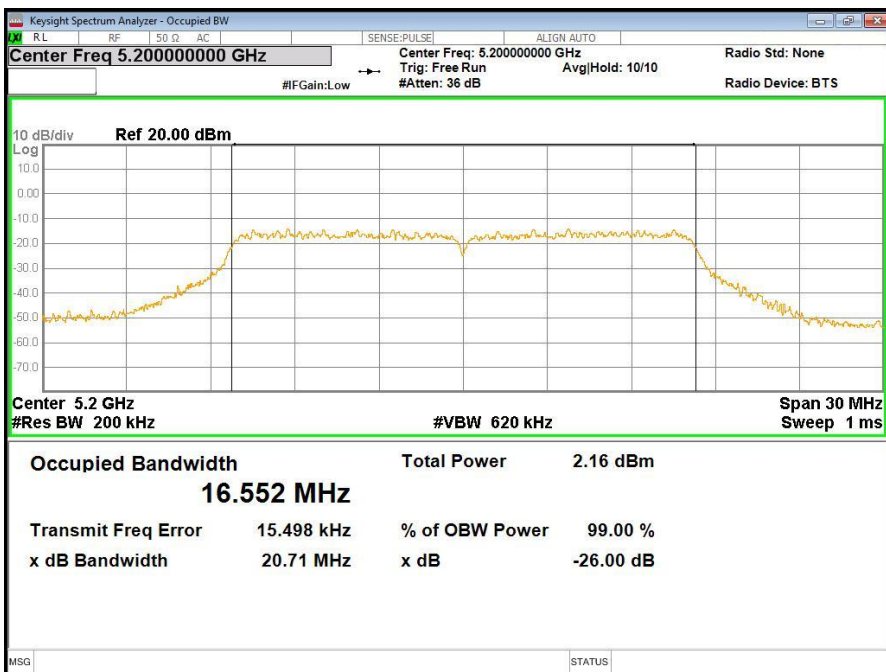
U-NII-1 11a Middle CH 5200MHZ
