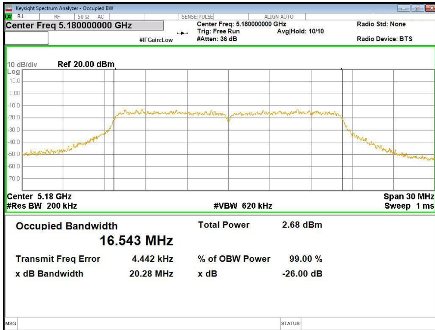
U-NII-1 11a Low CH 5180MHZ
