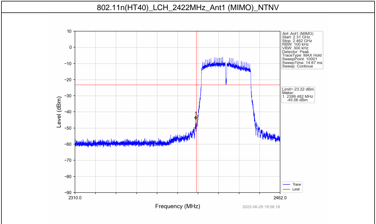
802.11n(HT40)_LCH_2422MHz_Ant1 (MIMO)_NTNV
