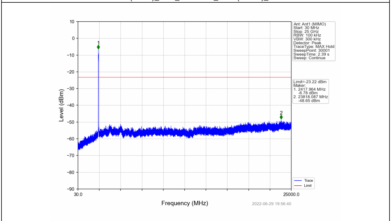
802.11n(HT40)_LCH_2422MHz_Ant1 (MIMO)_NTNV
