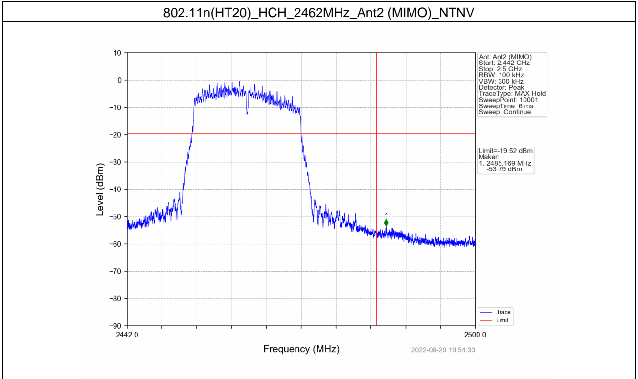
802.11n(HT20)_HCH_2462MHz_Ant2 (MIMO)_NTNV
