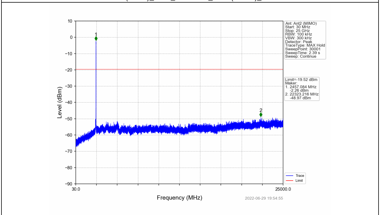
802.11n(HT20)_HCH_2462MHz_Ant2 (MIMO)_NTNV
