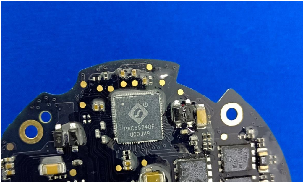
(13) EUT Photo
