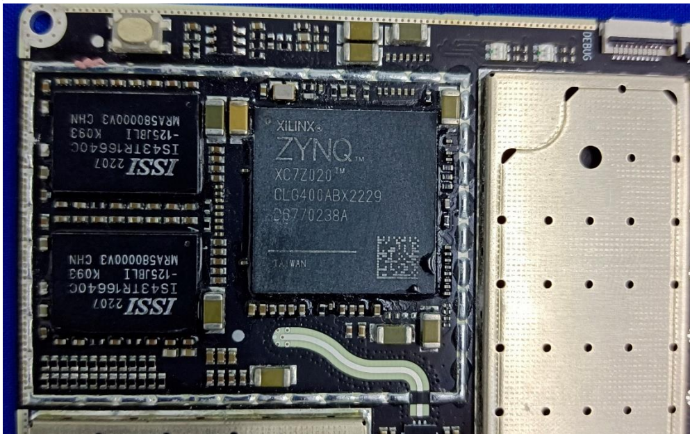
(14) EUT Photo
