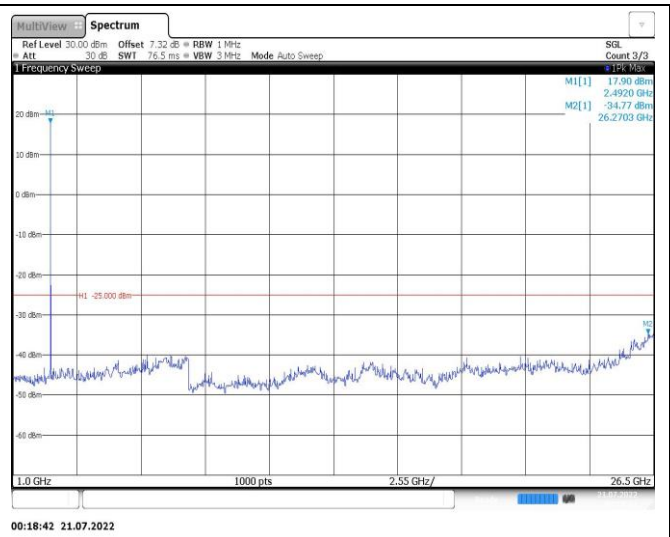
Band7-5MHz-QPSK-21100-1RB#0-Range2:1000~26500MHz
