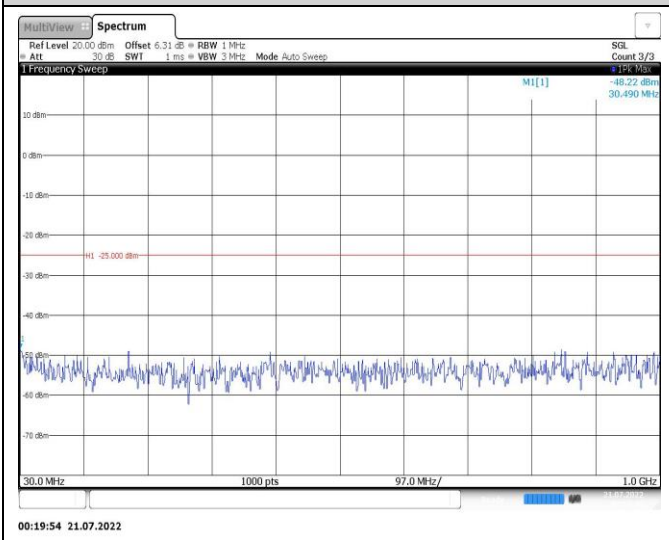
Band7-10MHz-QPSK-20800-1RB#0-Range1:30~1000MHz
