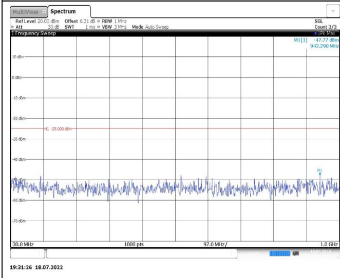
Band12-1.4MHz-QPSK-23017-1RB#0-Range1:30~1000MHz
