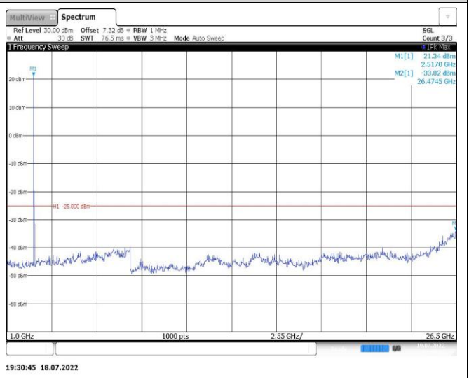
Band7-20MHz-QPSK-21350-1RB#0-Range2:1000~26500MHz
