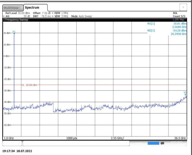
Band7-20MHz-QPSK-20850-1RB#0-Range2:1000~26500MHz
