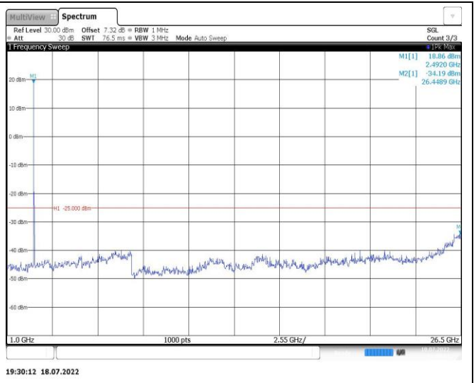
Band7-20MHz-QPSK-21100-1RB#0-Range2:1000~26500MHz
