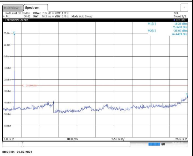
Band7-10MHz-QPSK-20800-1RB#0-Range2:1000~26500MHz
