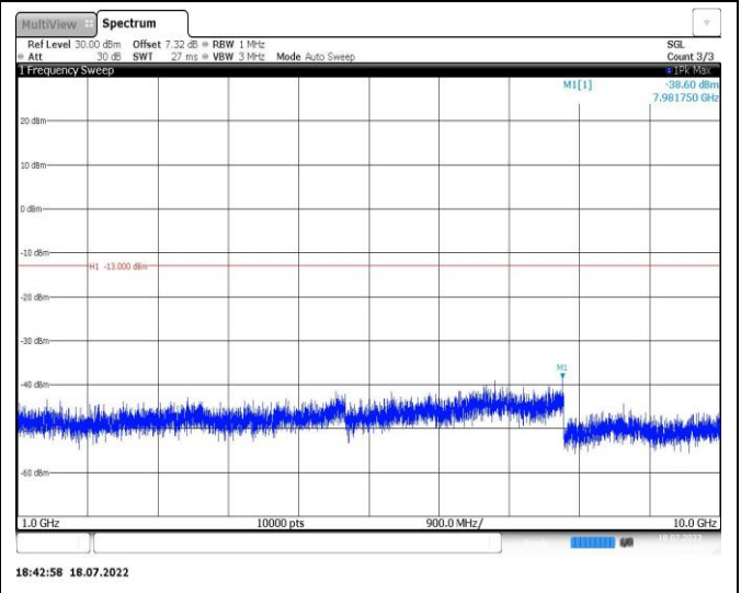
Band5-3MHz-QPSK-20635-1RB#0-Range2:1000~10000MHz
