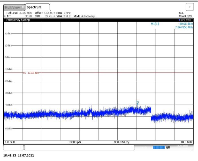
Band5-3MHz-QPSK-20415-1RB#0-Range2:1000~10000MHz
