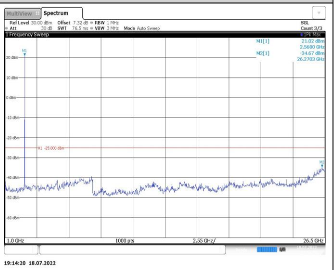
Band7-15MHz-QPSK-20825-1RB#0-Range2:1000~26500MHz
