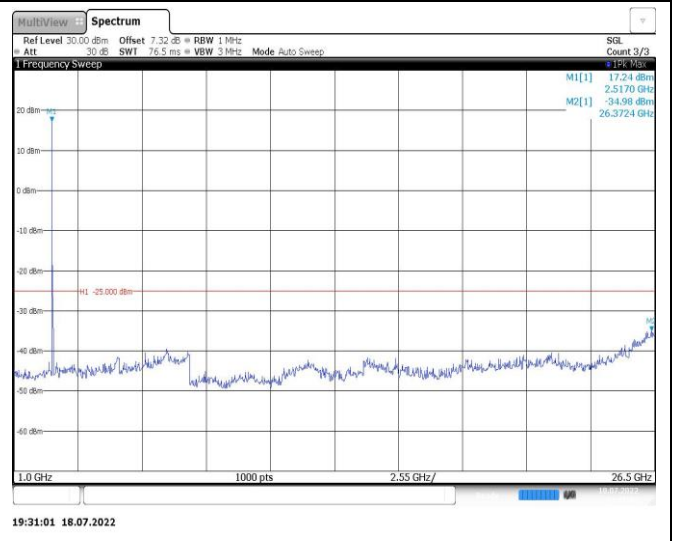
Band7-20MHz-16QAM-21350-1RB#0-Range2:1000~26500MHz
