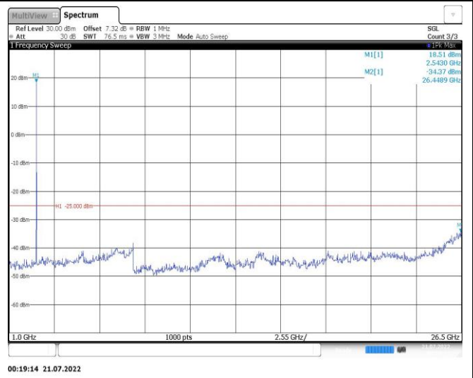
Band7-5MHz-QPSK-21425-1RB#0-Range2:1000~26500MHz
