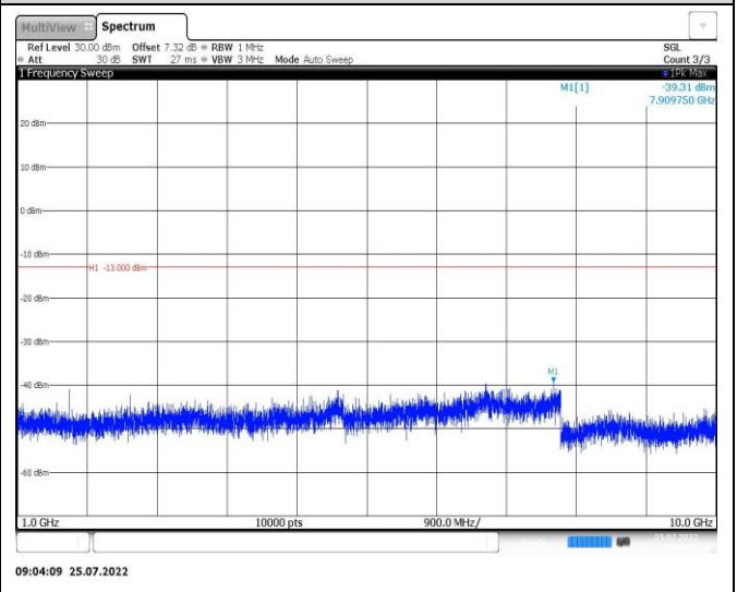
Band26-10MHz-QPSK-26990-1RB#0-Range2:1000~10000MHz
