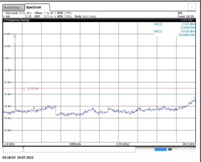
Band38-20MHz-QPSK-37850-1RB#0-Range2:1000~26500MHz
