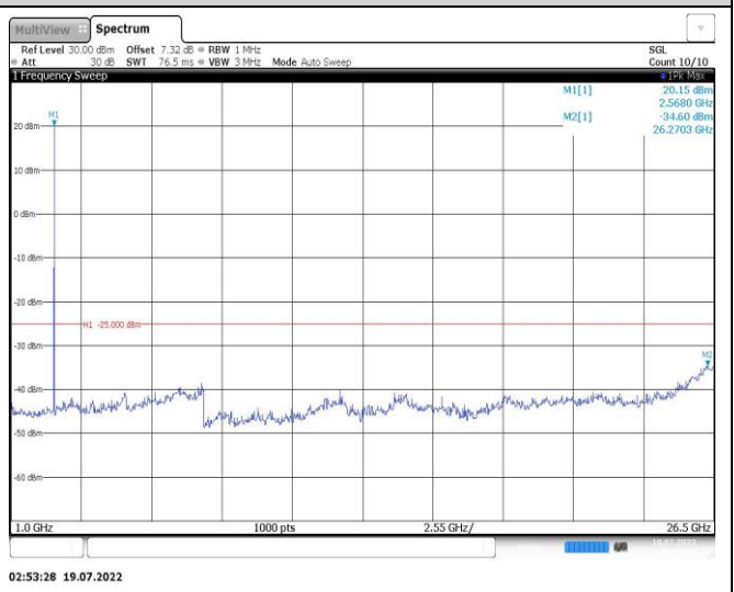
Band38-5MHz-QPSK-38000-1RB#0-Range2:1000~26500MHz
