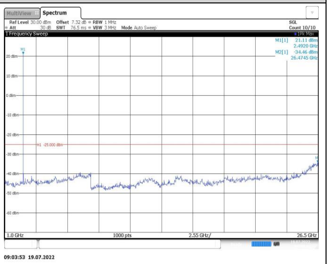
Band41-5MHz-QPSK-40620-1RB#0-Range2:1000~26500MHz
