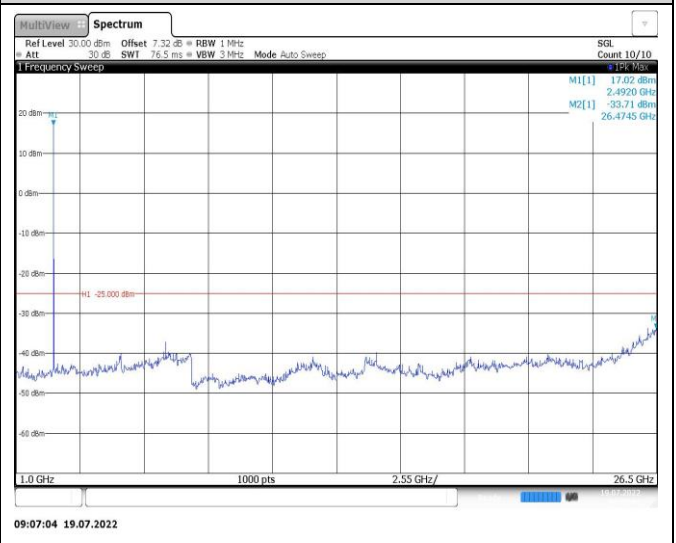
Band41-10MHz-QPSK-40620-1RB#0-Range2:1000~26500MHz
