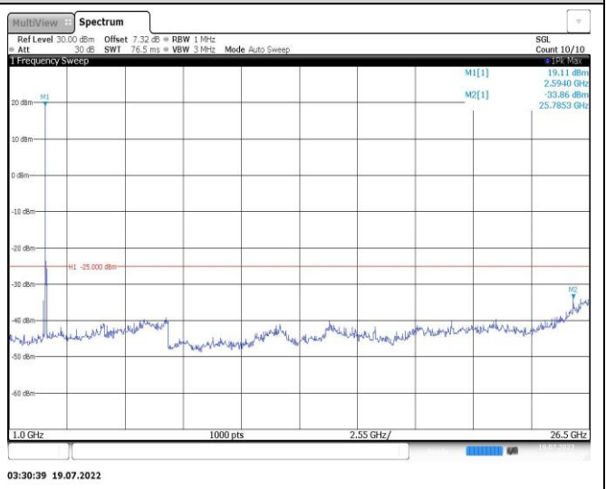
Band38-20MHz-16QAM-37850-1RB#0-Range2:1000~26500MHz
