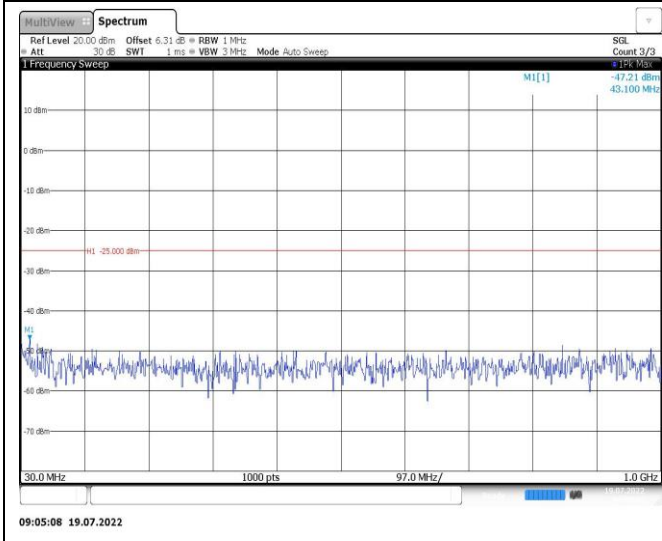
Band41-10MHz-QPSK-39700-1RB#0-Range1:30~1000MHz
