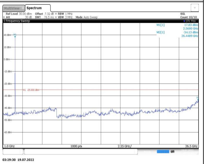
Band38-20MHz-QPSK-38000-1RB#0-Range2:1000~26500MHz
