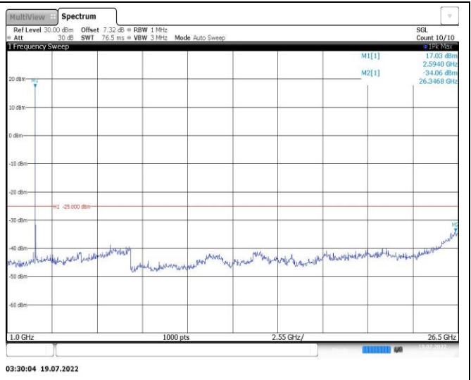
Band38-20MHz-QPSK-38150-1RB#0-Range2:1000~26500MHz
