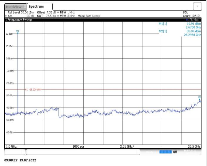
Band41-15MHz-QPSK-39725-1RB#0-Range2:1000~26500MHz
