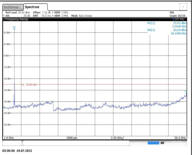
Band41-5MHz-QPSK-39675-1RB#0-Range2:1000~26500MHz
