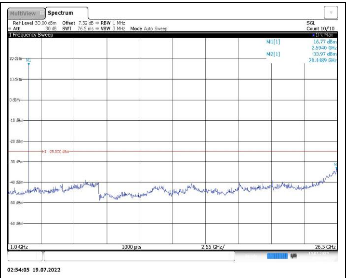
Band38-5MHz-QPSK-38225-1RB#0-Range2:1000~26500MHz
