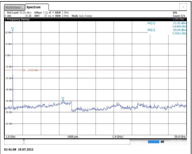
Band25-20MHz-16QAM-26365-1RB#0-Range2:1000~20000MHz
