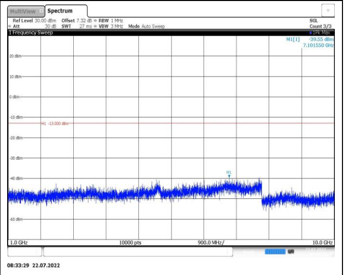
Band26-3MHz-QPSK-27025-1RB#0-Range2:1000~10000MHz
