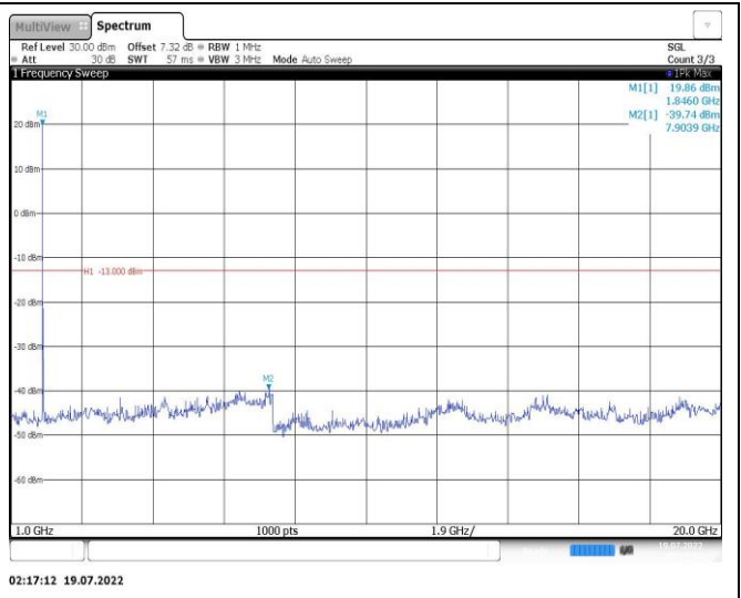
Band25-10MHz-16QAM-26365-1RB#0-Range2:1000~20000MHz
