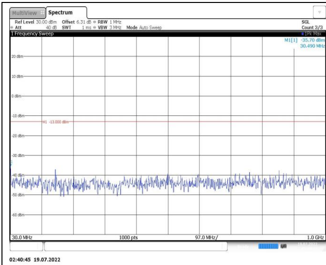
Band25-20MHz-QPSK-26365-1RB#0-Range1:30~1000MHz
