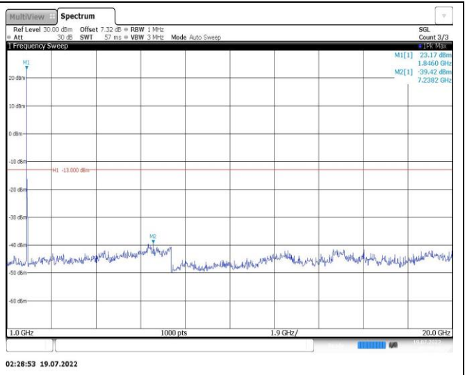
Band25-15MHz-QPSK-26365-1RB#0-Range2:1000~20000MHz
