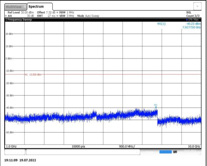
Band26-5MHz-QPSK-26765-1RB#0-Range2:1000~10000MHz
