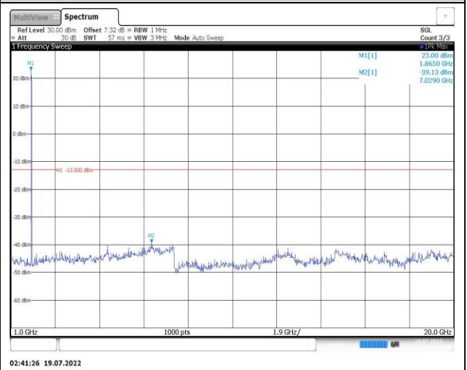
Band25-20MHz-QPSK-26590-1RB#0-Range2:1000~20000MHz
