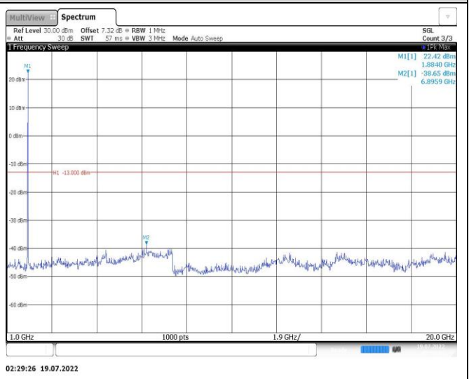
Band25-15MHz-QPSK-26615-1RB#0-Range2:1000~20000MHz
