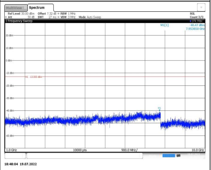
Band26-1.4MHz-QPSK-26797-1RB#0-Range2:1000~10000MHz
