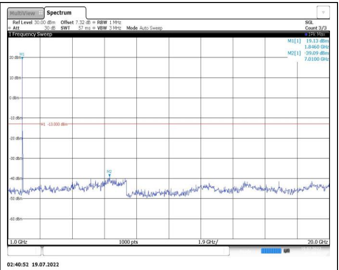
Band25-20MHz-QPSK-26365-1RB#0-Range2:1000~20000MHz
