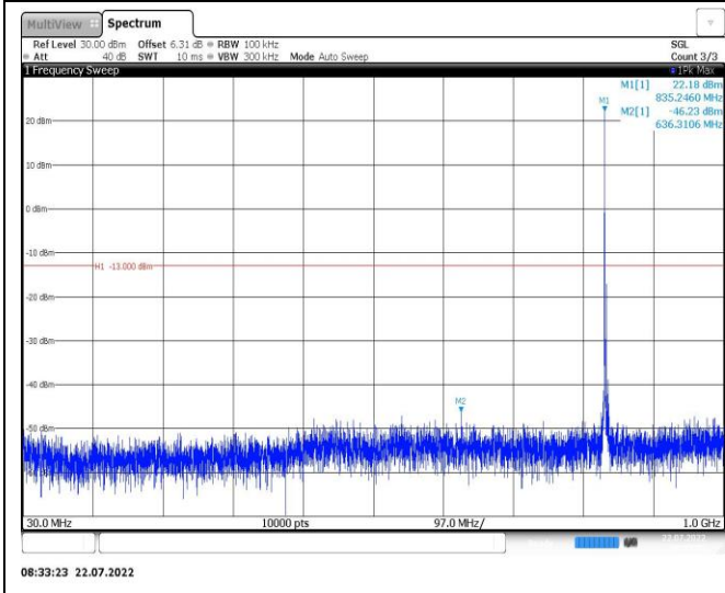
Band26-3MHz-QPSK-27025-1RB#0-Range1:30~1000MHz
