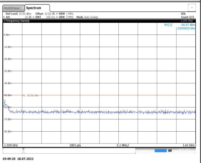
Band13-5MHz-QPSK-23255-1RB#0-Range2:1000~10000MHz
