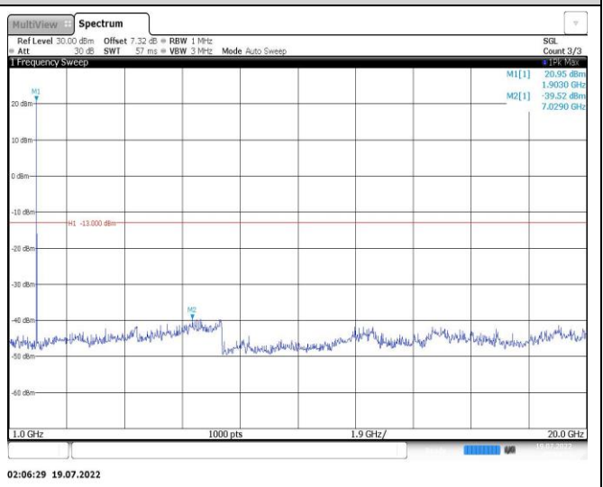
Band25-10MHz-QPSK-26090-1RB#0-Range2:1000~20000MHz
