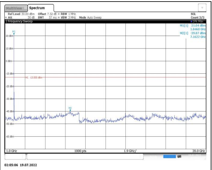
Band25-5MHz-QPSK-26365-1RB#0-Range2:1000~20000MHz
