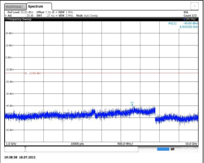
Band12-3MHz-QPSK-23165-1RB#0-Range2:1000~10000MHz
