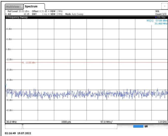
Band25-10MHz-QPSK-26365-1RB#0-Range1:30~1000MHz
