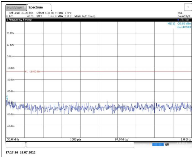
Band2-20MHz-QPSK-18900-1RB#0-Range1:30~1000MHz
