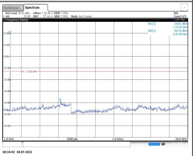
Band4-5MHz-QPSK-19975-1RB#0-Range2:1000~20000MHz
