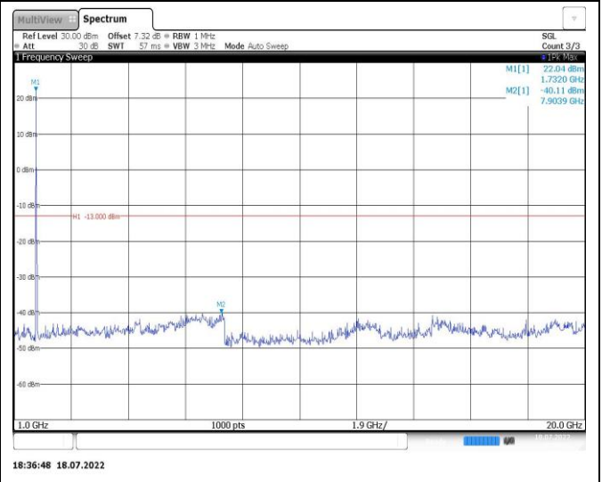
Band4-20MHz-QPSK-20300-1RB#0-Range2:1000~20000MHz
