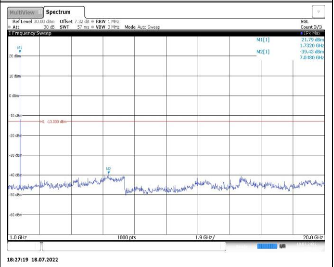
Band4-5MHz-QPSK-20375-1RB#0-Range2:1000~20000MHz
