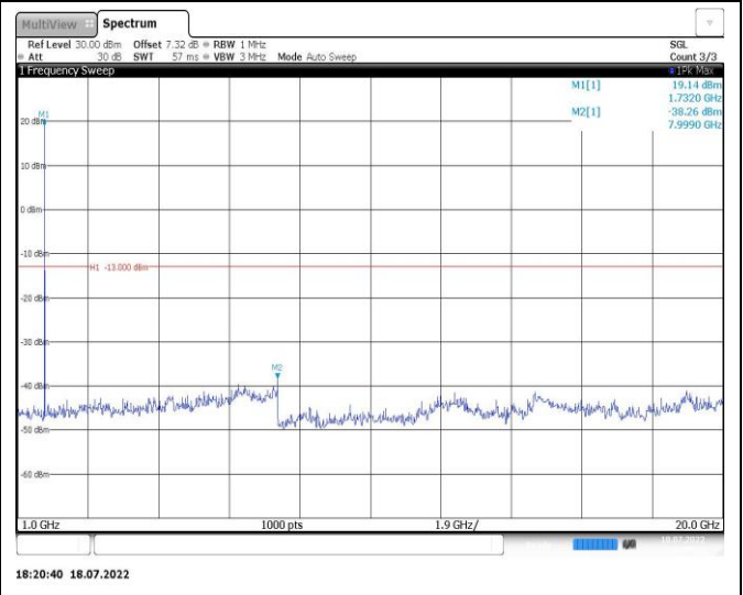
Band4-1.4MHz-QPSK-20393-1RB#0-Range2:1000~20000MHz
