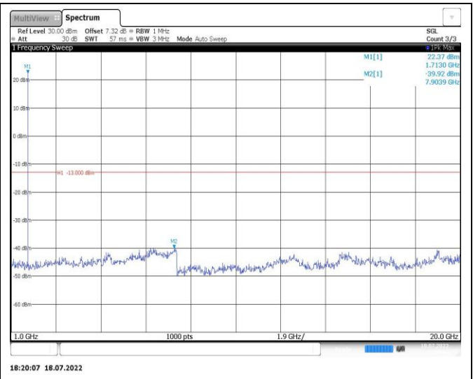
Band4-1.4MHz-QPSK-20175-1RB#0-Range2:1000~20000MHz
