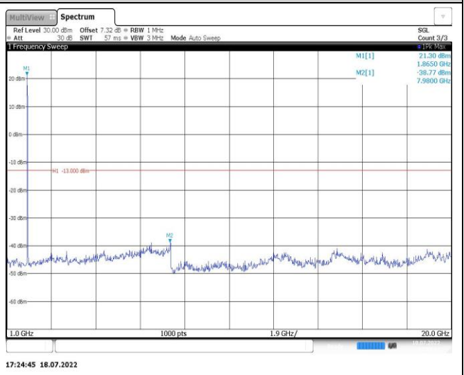
Band2-15MHz-QPSK-19125-1RB#0-Range2:1000~20000MHz
