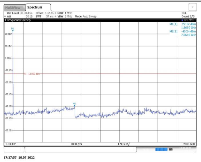
Band2-20MHz-QPSK-19100-1RB#0-Range2:1000~20000MHz
