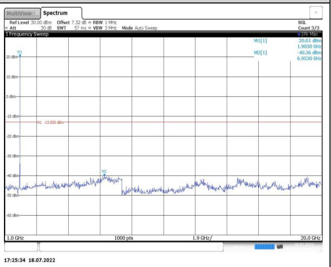
Band2-20MHz-QPSK-18700-1RB#0-Range2:1000~20000MHz
