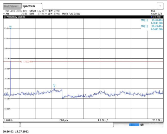
Band2-3MHz-QPSK-19185-1RB#0-Range2:1000~20000MHz
