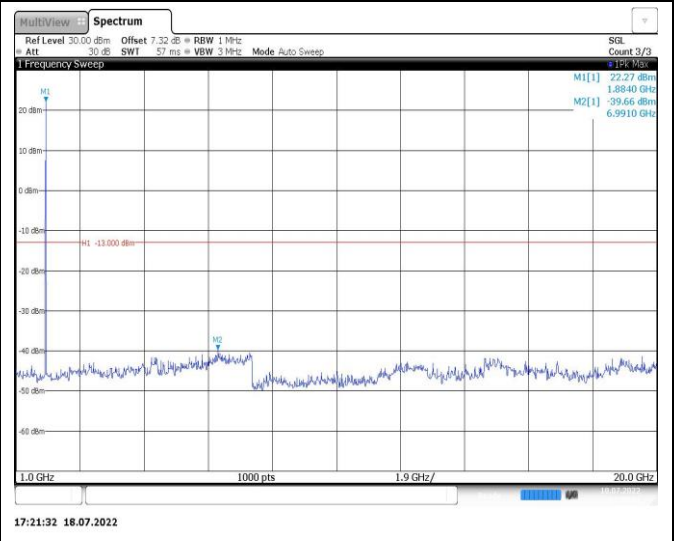
Band2-10MHz-QPSK-19150-1RB#0-Range2:1000~20000MHz
