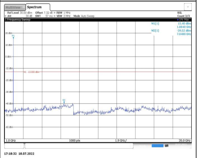
Band2-5MHz-16QAM-19175-1RB#0-Range2:1000~20000MHz
