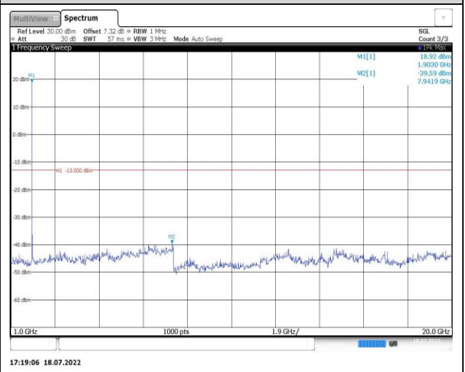
Band2-10MHz-QPSK-18650-1RB#0-Range2:1000~20000MHz
