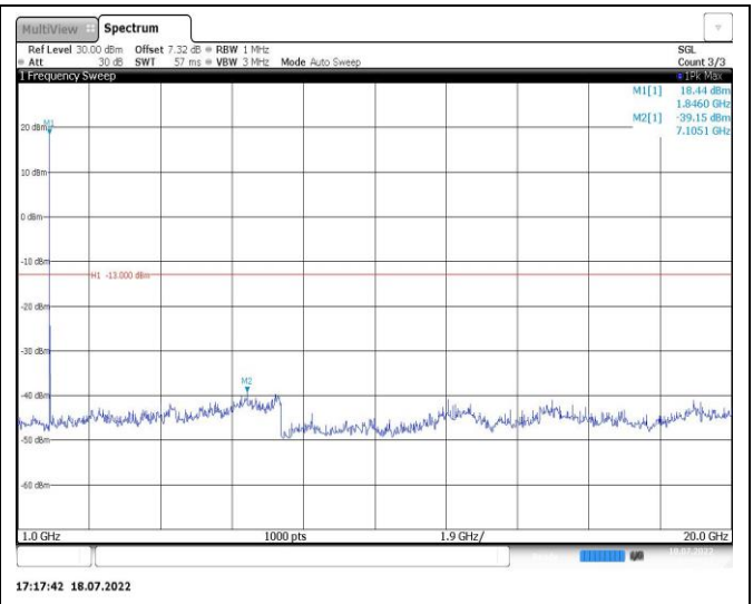
Band2-5MHz-QPSK-18900-1RB#0-Range2:1000~20000MHz
