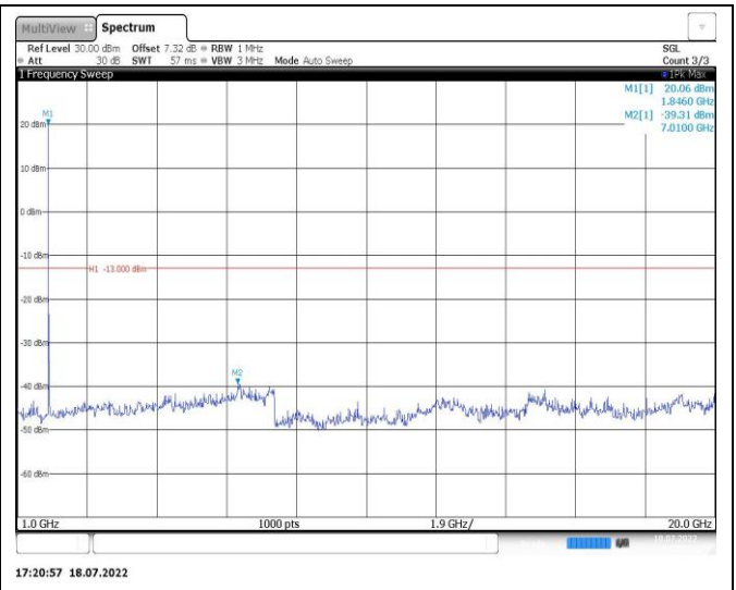
Band2-10MHz-QPSK-18900-1RB#0-Range2:1000~20000MHz
