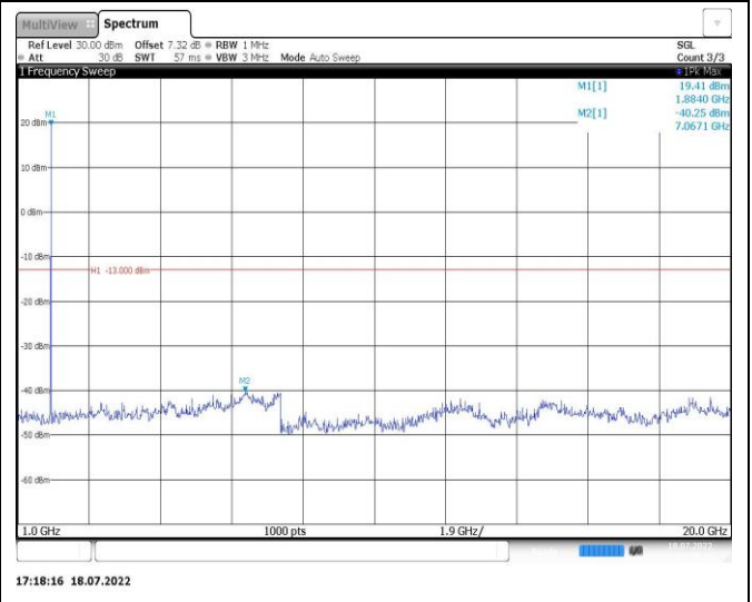
Band2-5MHz-QPSK-19175-1RB#0-Range2:1000~20000MHz
