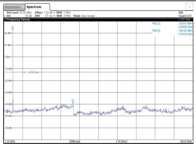
Band2-1.4MHz-QPSK-19193-1RB#0-Range2:1000~20000MHz
