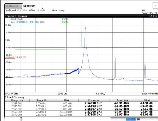
Band38-20MHz-QPSK-37850-1RB#0
