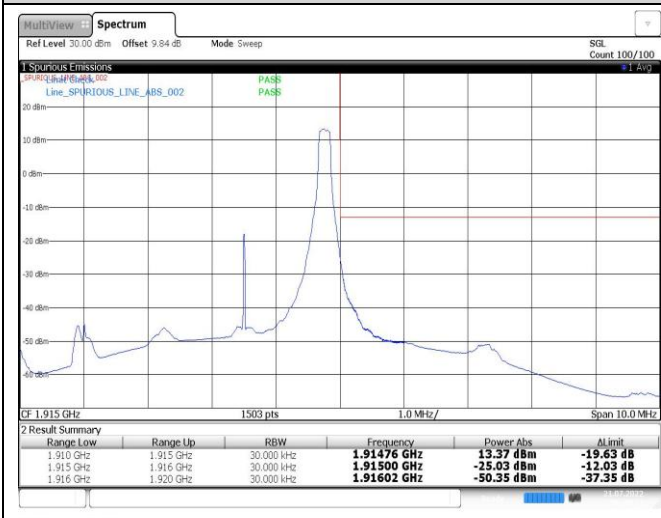
Band25-3MHz-QPSK-26675-1RB#14
