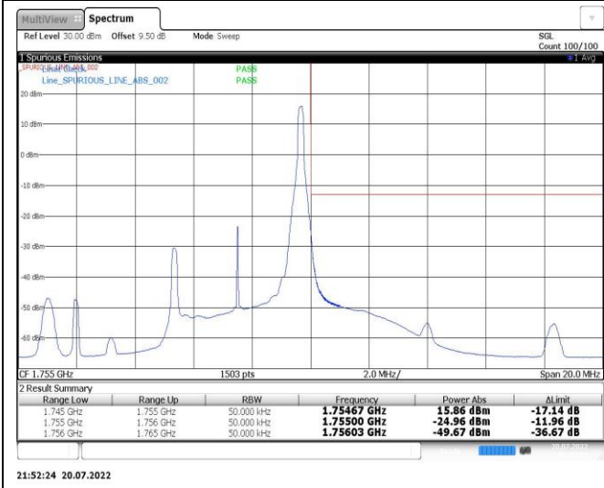
Band4-10MHz-QPSK-20000-1RB#0
