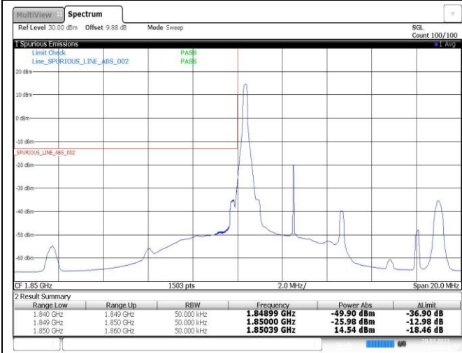
Band2-5MHz-16QAM-18625-1RB#0
