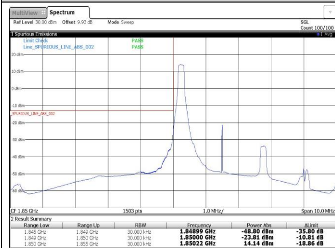
Band2-3MHz-QPSK-18615-1RB#0
