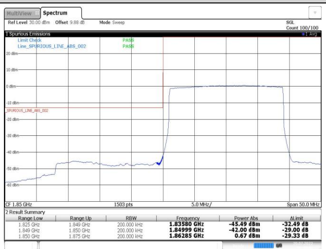
Band2-20MHz-QPSK-18700-100RB#0
