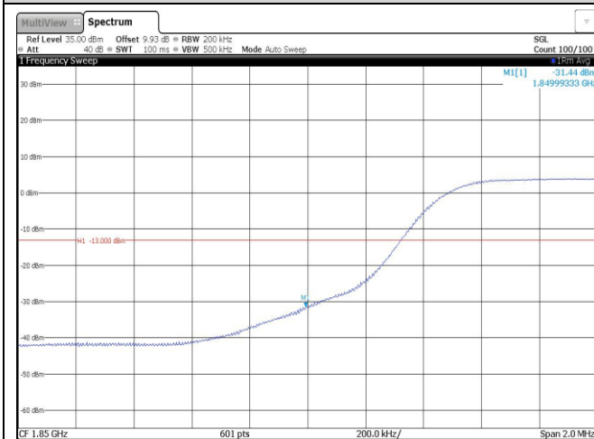
Band2-10MHz-QPSK-18650-50RB#0
