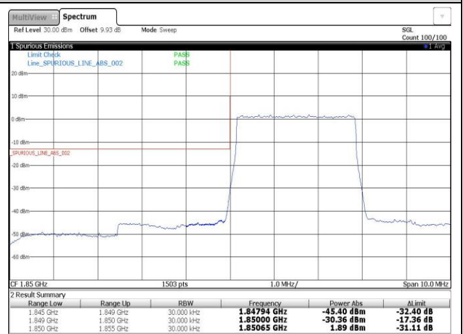
Band2-3MHz-QPSK-18615-15RB#0
