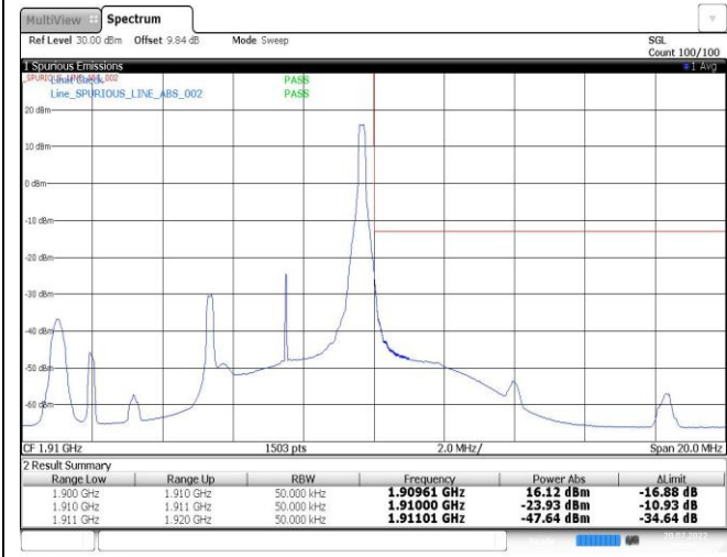
Band2-5MHz-QPSK-19175-1RB#24
