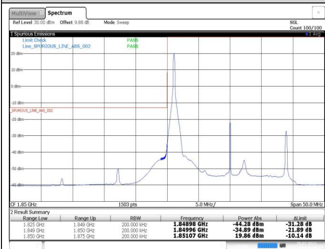
Band2-20MHz-QPSK-18700-1RB#0
