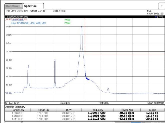
Band2-15MHz-16QAM-19125-1RB#74
