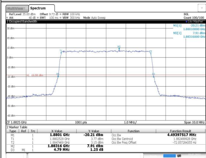
Band25-5MHz-QPSK-26365-25RB#0
