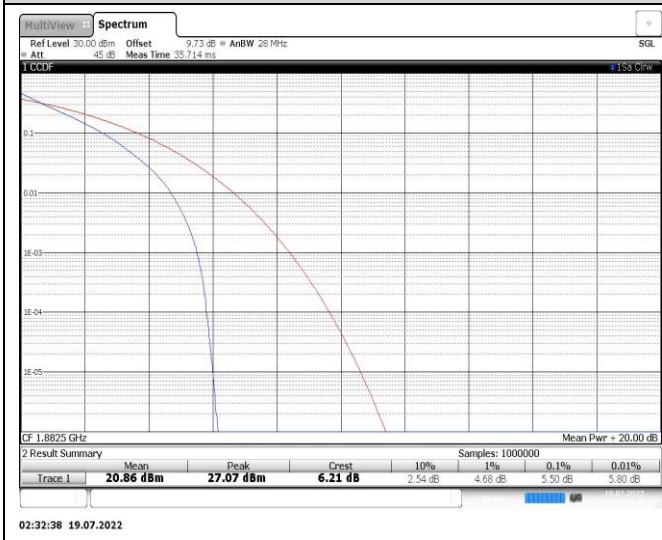
Band25-20MHz-QPSK-26365-100RB#0
