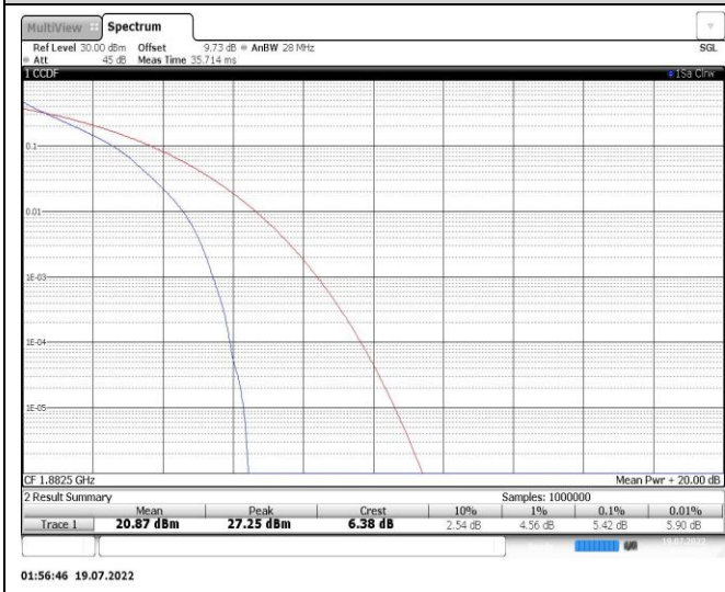
Band25-5MHz-QPSK-26365-25RB#0
