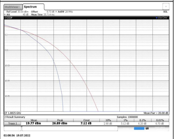
Band25-10MHz-16QAM-26365-50RB#0
