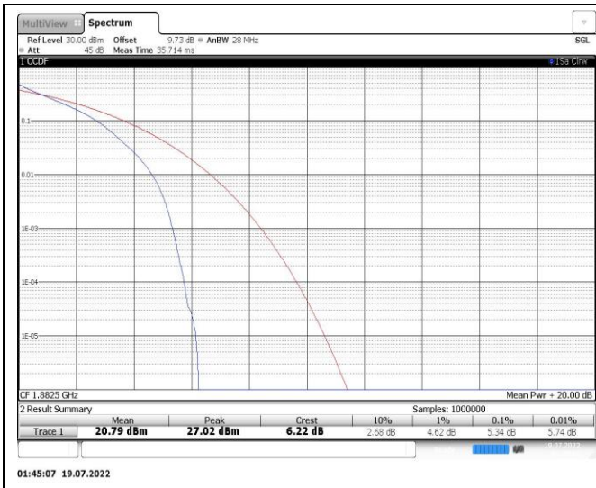
Band25-3MHz-QPSK-26365-15RB#0
