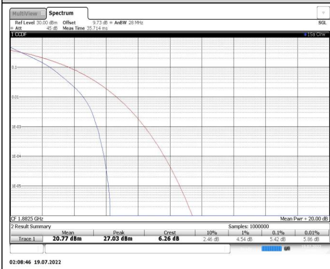
Band25-10MHz-QPSK-26365-50RB#0
