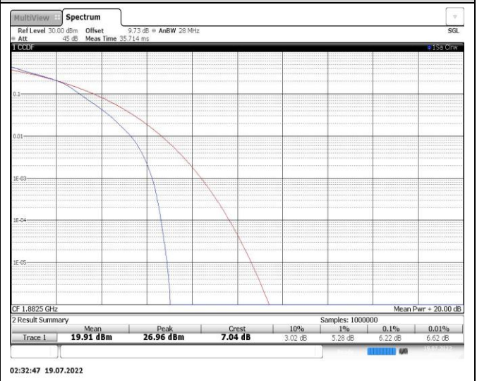
Band25-20MHz-16QAM-26365-100RB#0
