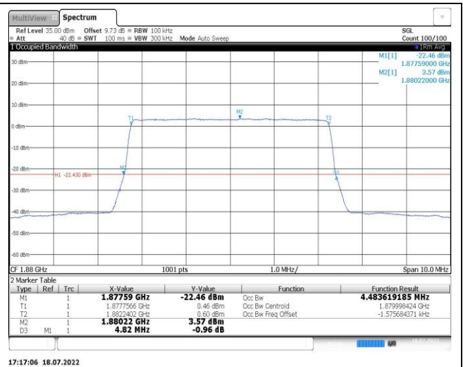
Band2-10MHz-16QAM-18900-50RB#0
