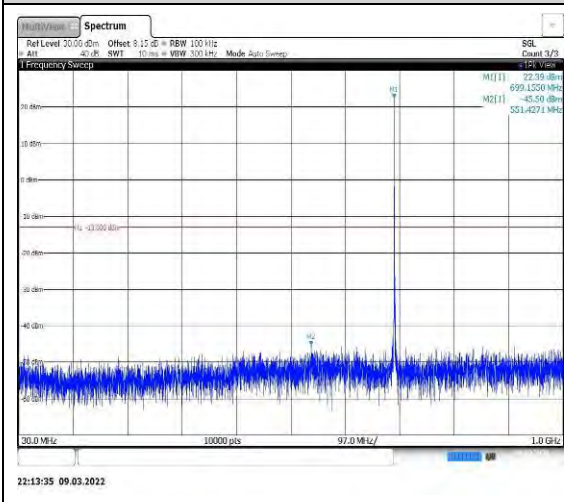
Band12-1.4MHz-QPSK-23017-1RB#0-Range 1:30~1000MHz
