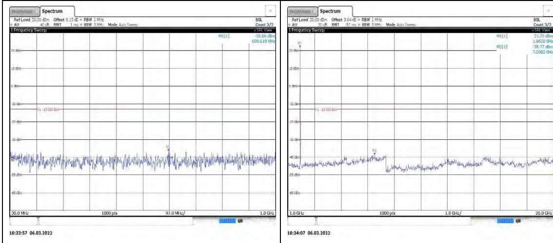
Band2-20MHz-16QAM-18900-1RB#0-Range 1:30~1000MHz 2:1000~20000MHz
