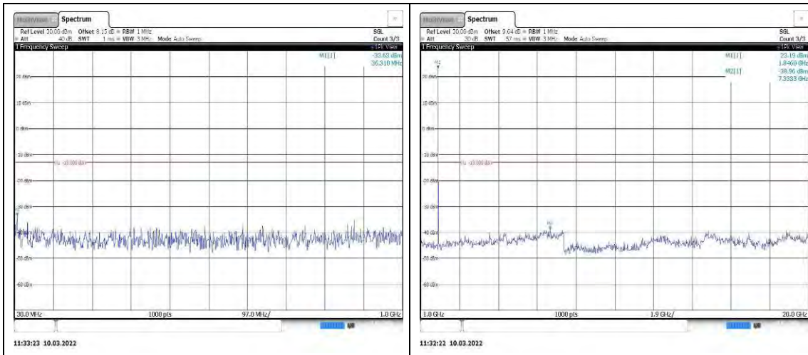
Band25-20MHz-QPSK-26590-1RB#0-Range 1:30~1000MHz Band25-20MHz-16QAM-26140-1RB#0-Rang e2:1000~20000MHz
