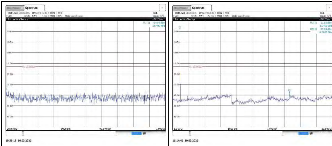
Band25-10MHz-16QAM-26640-1RB#0-Rang e1:30~1000MHz
