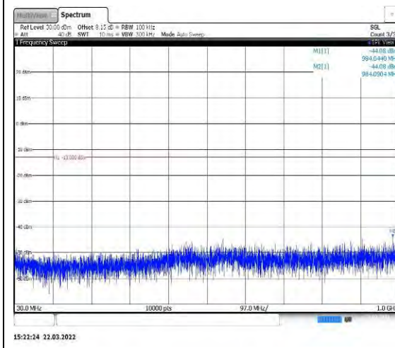
Band13-5MHz-QPSK-23255-1RB#0-Range1: 30~1000MHz
