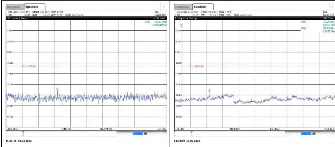
Band25-20MHz-16QAM-26140-1RB#0-Rang e1:30~1000MHz Band25-20MHz-16QAM-26365-1RB#0-Rang e2:1000~20000MHz
