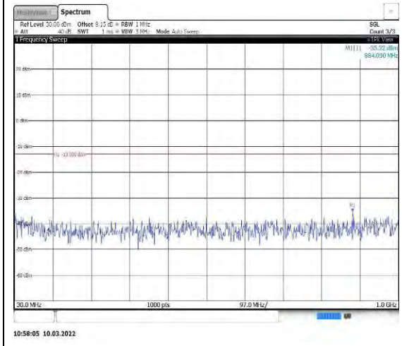
Band25-10MHz-QPSK-26365-1RB#0-Range 1:30~1000MHz
