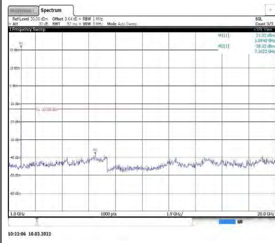
Band25-3MHz-QPSK-26365-1RB#0-Range2: 1000~20000MHz
