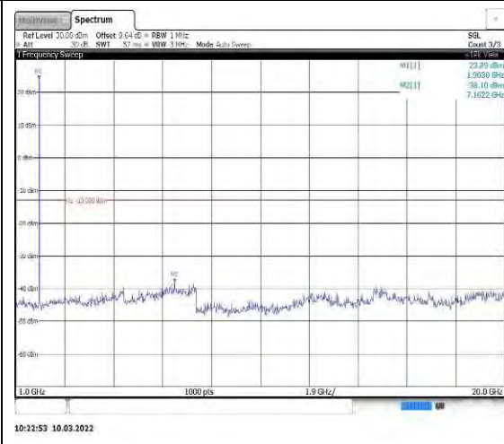
Band25-3MHz-QPSK-26675-1RB#0-Range2: 1000~20000MHz
