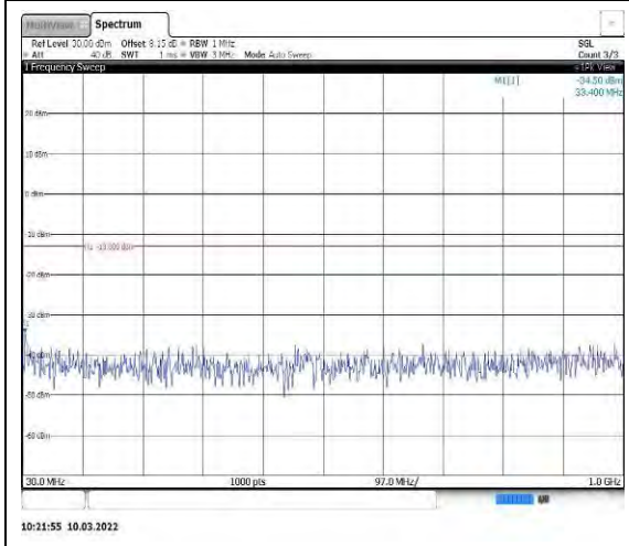
Band25-3MHz-QPSK-26365-1RB#0-Range1: 30~1000MHz
