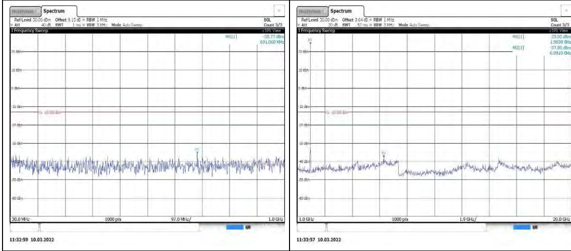
Band25-20MHz-16QAM-26365-1RB#0-Rang e1:30~1000MHz Band25-20MHz-16QAM-26590-1RB#0-Rang e2:1000~20000MHz
