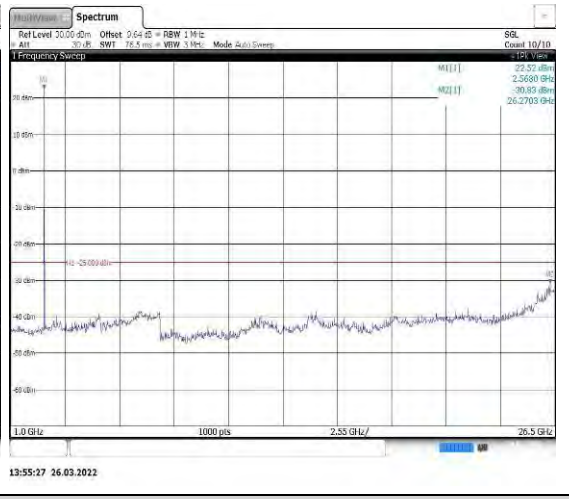
Band38-10MHz-QPSK-37800-1RB#0-Range2: 1000~26500MHz
