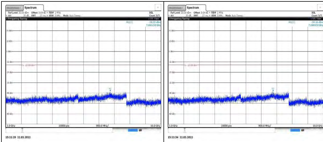
Band13-5MHz-QPSK-23230-1RB#0-Range2: 1000~10000MHz
