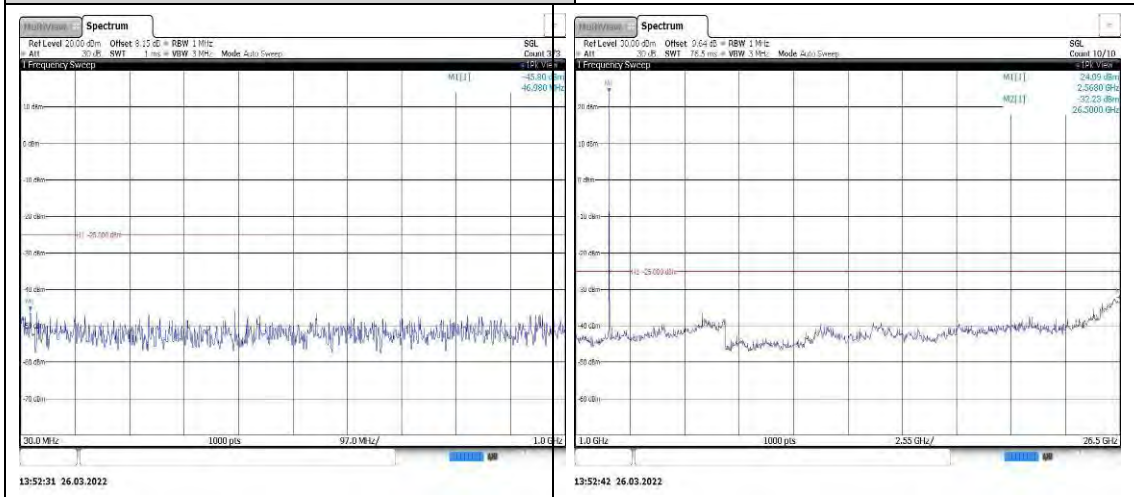
Band38-5MHz-QPSK-37775-1RB#0-Range 1:30~1000MHz Band38-5MHz-QPSK-37775-1RB#0-Range2:1 000~26500MHz
