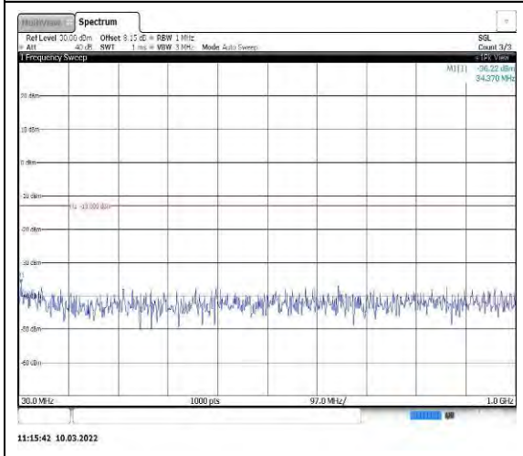
Band25-15MHz-16QAM-26365-1RB#0-Rang e1:30~1000MHz
