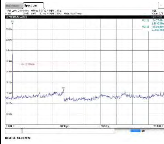
Band25-10MHz-QPSK-26365-1RB#0-Range 2:1000~20000MHz
