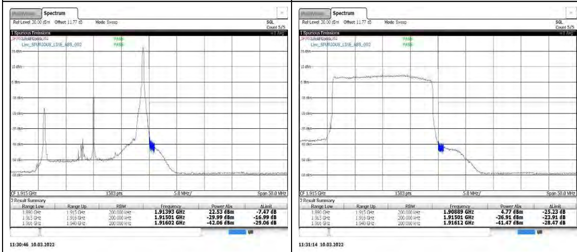
Band25-20MHz-16QAM-26590-1RB#99
